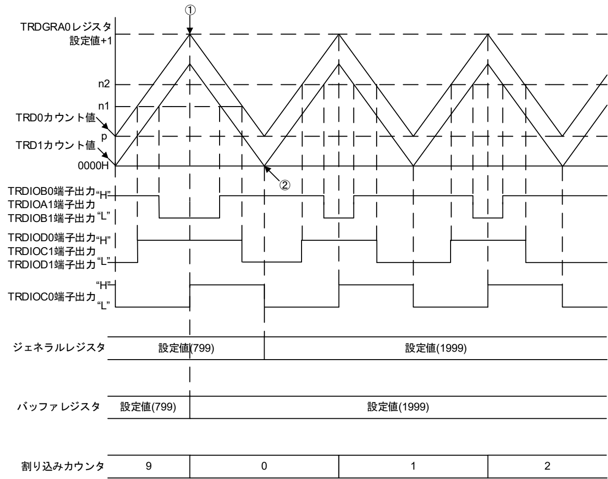
PWM波形1→PWM波形2
