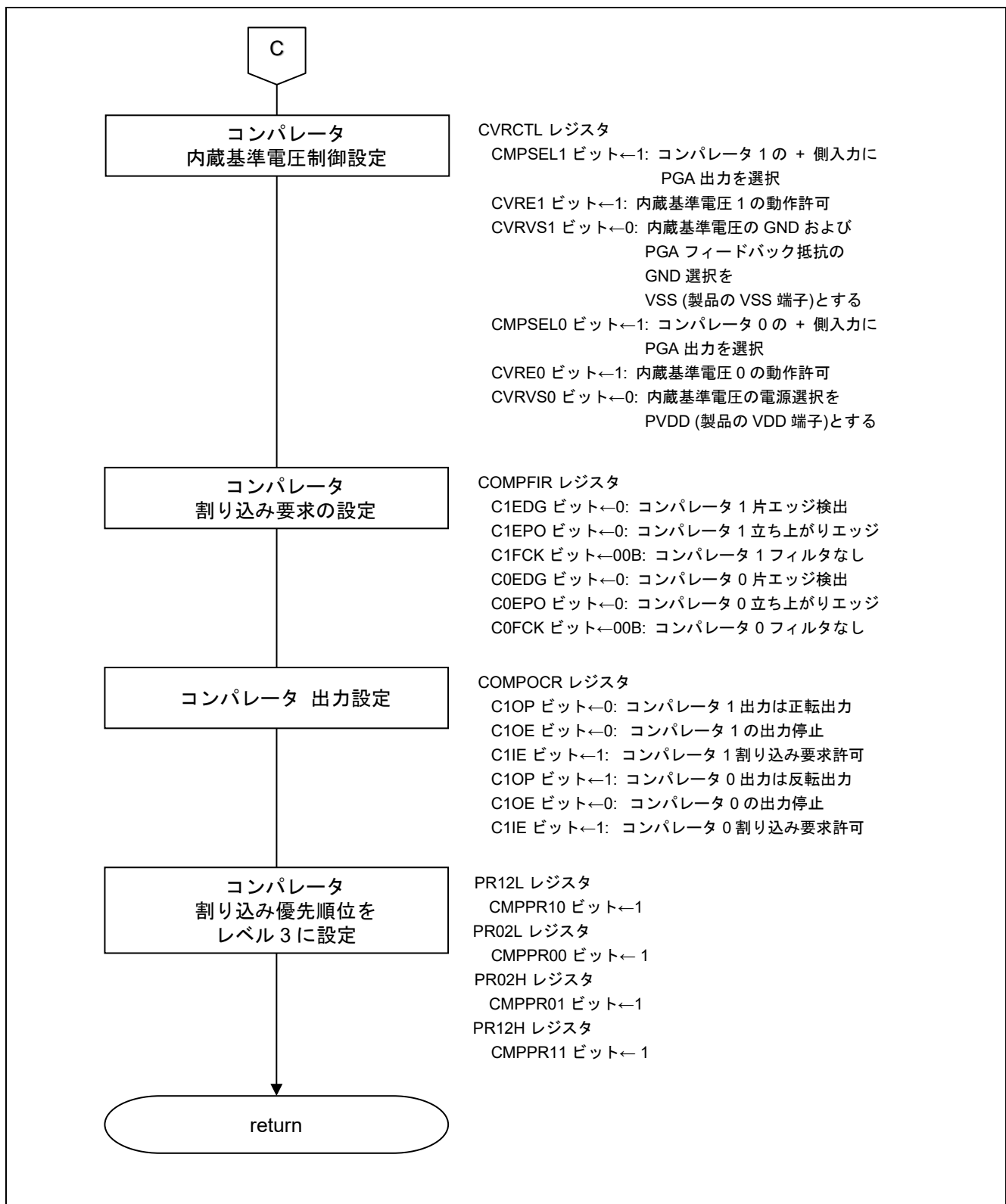
図 4.20 コンパレータ・PGA 初期設定(2/2)
