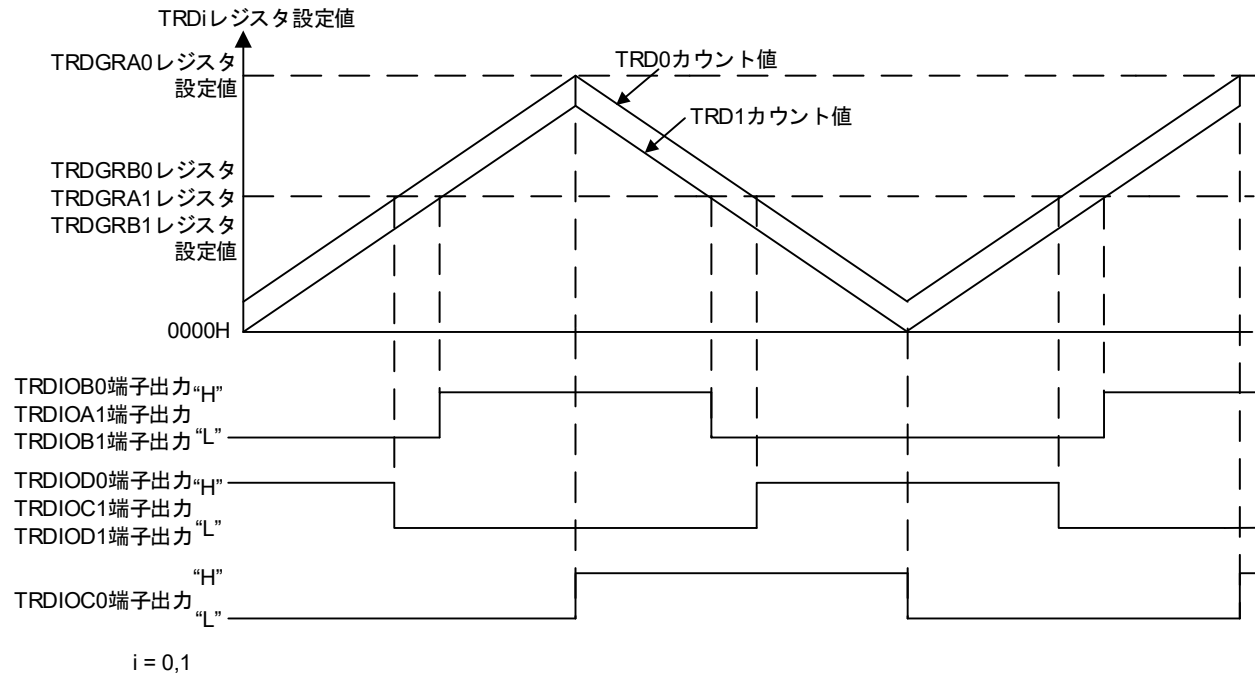
図 1.3 相補 PWM の出力波形
