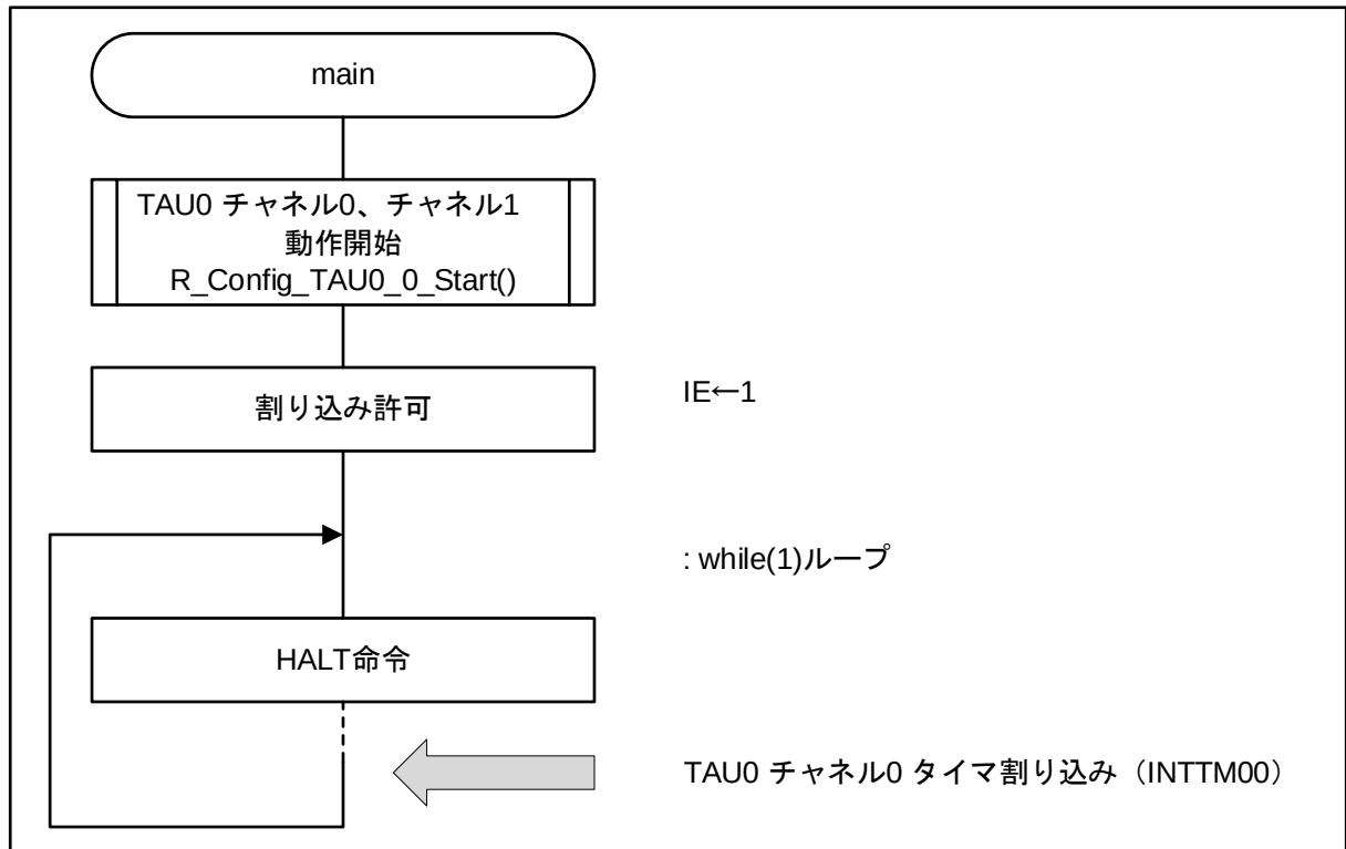
図 4-1 メイン処理
