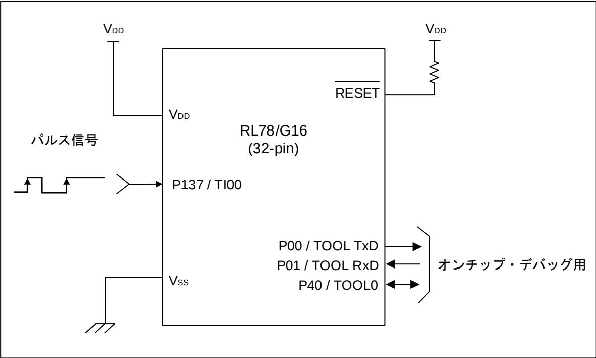
図 3-1 ハードウェア構成
