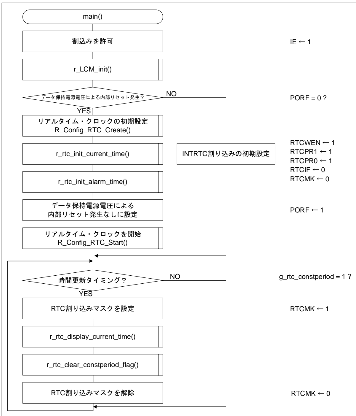
図 4-1 メイン処理
