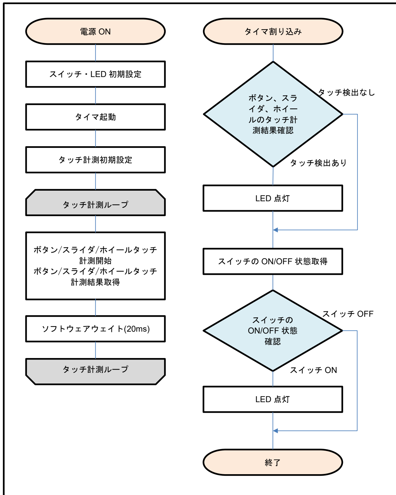
図 3-5 処理フロー（自己容量タッチボタン／ホイール／スライダボード）
