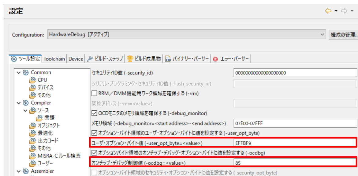
図 3-4 ユーザ・オプション・バイト値およびオンチップ・デバッグ制御値
