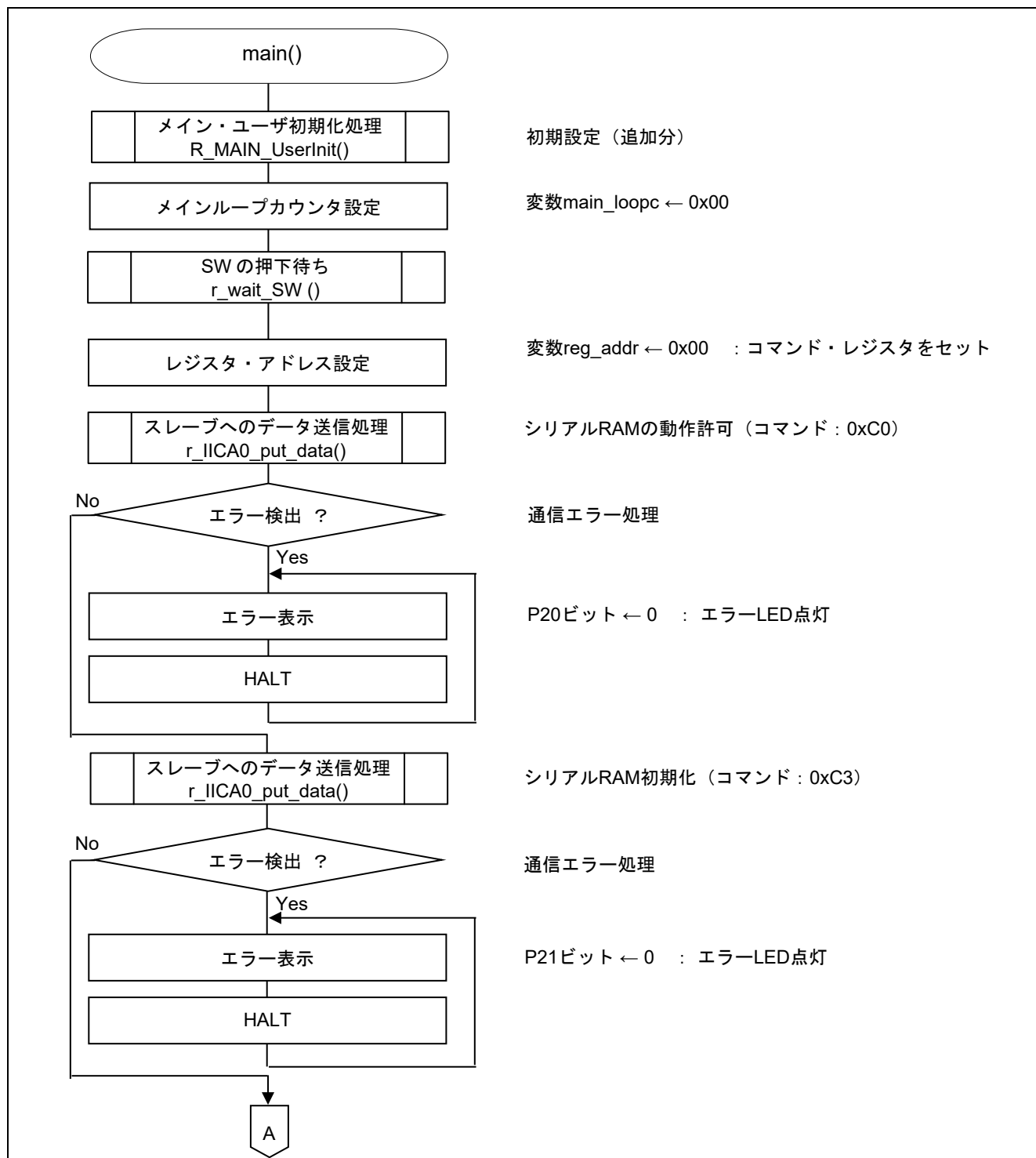
図 5.1 メイン処理 (1/3)
