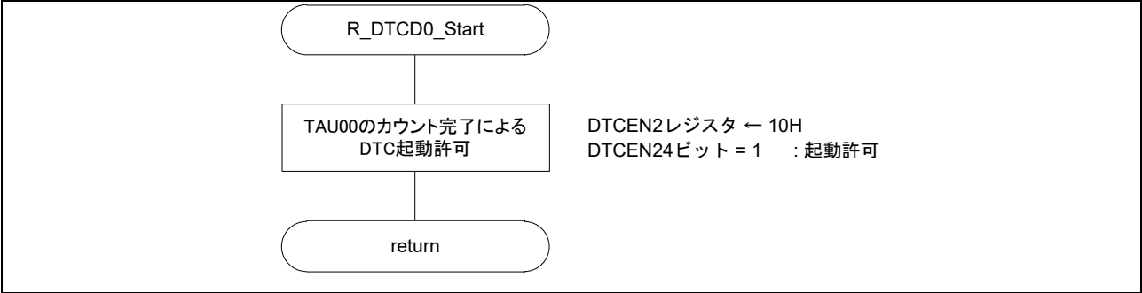
図 4.12 DTC 起動
