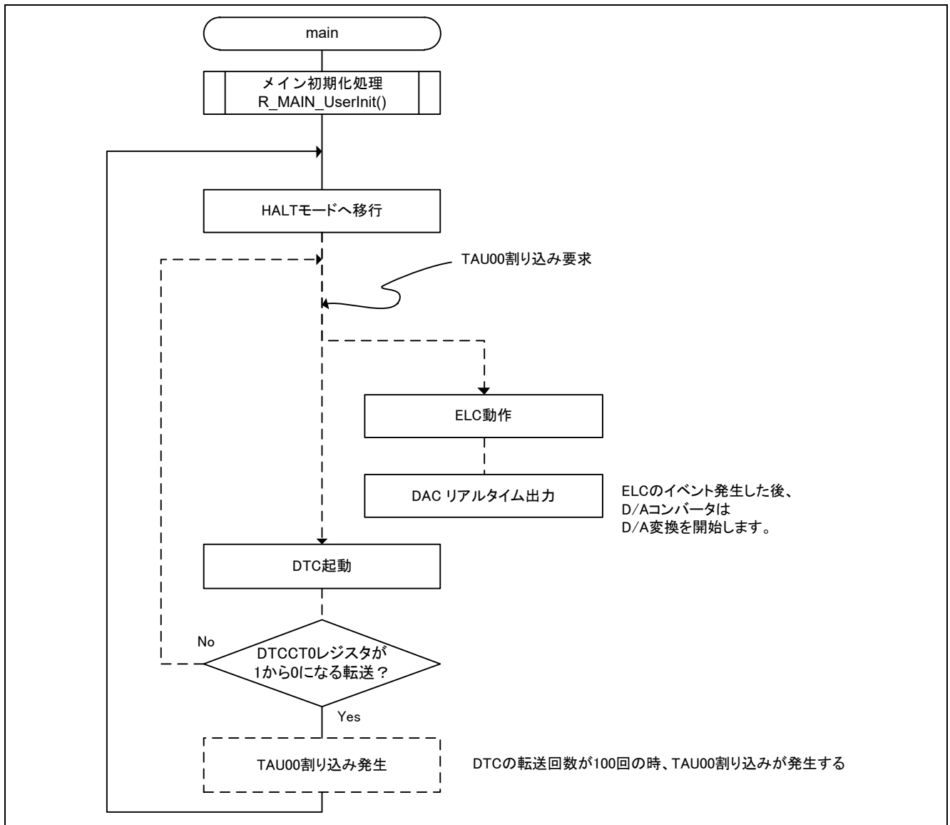
図 4.10 メイン処理
