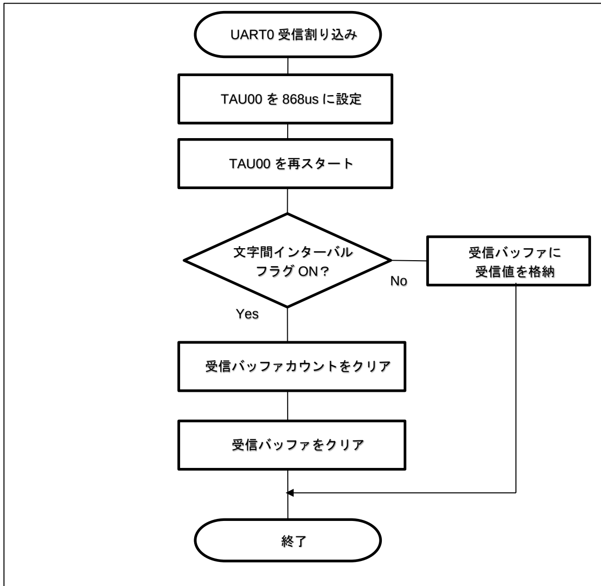
図 5-6 シリアル受信割り込み処理（スレーブモード（RTU））
