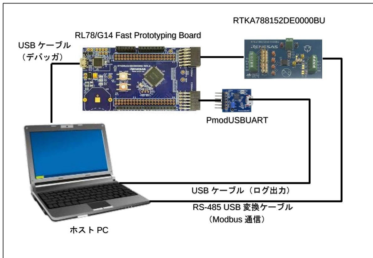
図 4-1 RL78 – PC(GUI)環境の構成例
