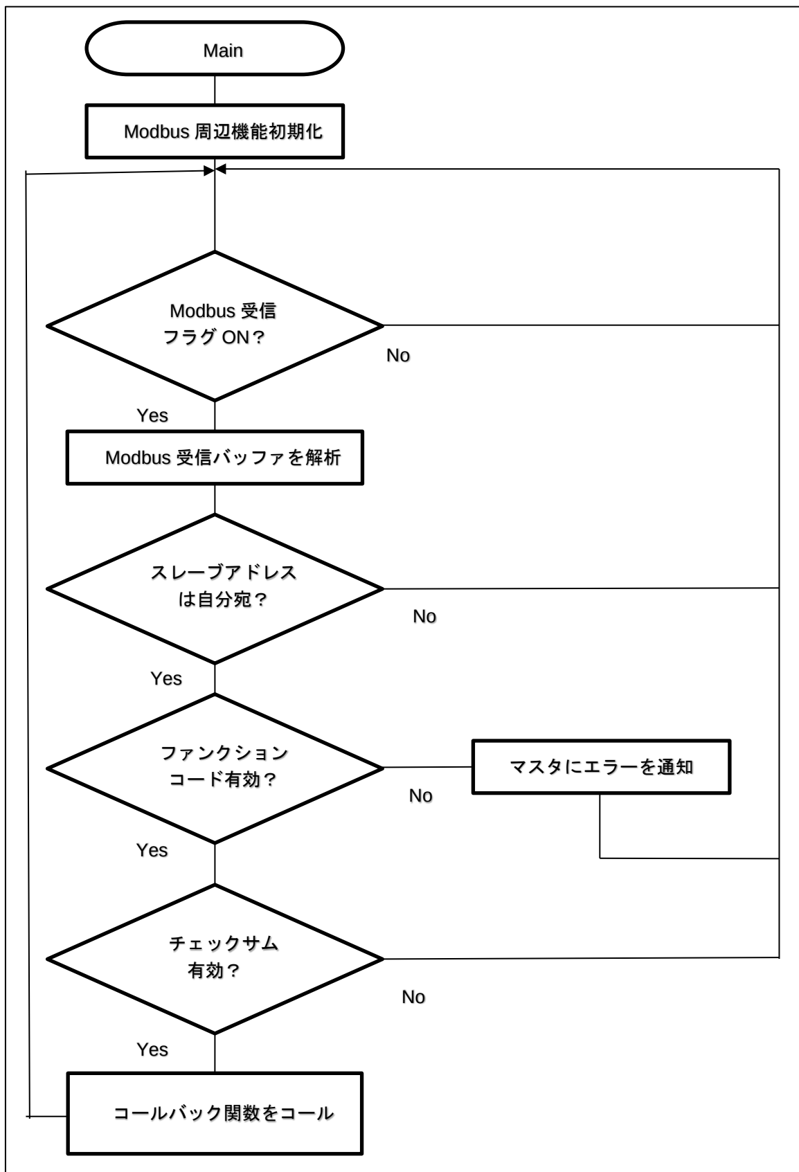
図 5-2 メイン処理（スレーブモード（ASCII））
