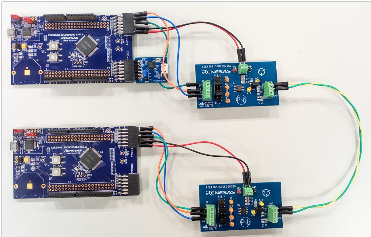
図 6-2 ボード接続写真
