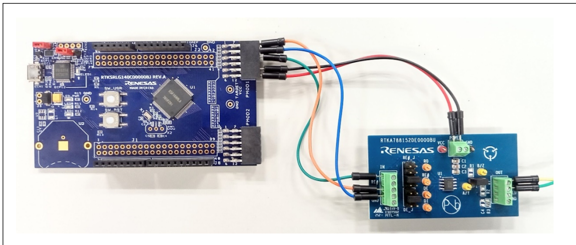
図 4-4 RL78/G14 Fast Prototyping Board - RTKA788152DE0000BU 接続写真
