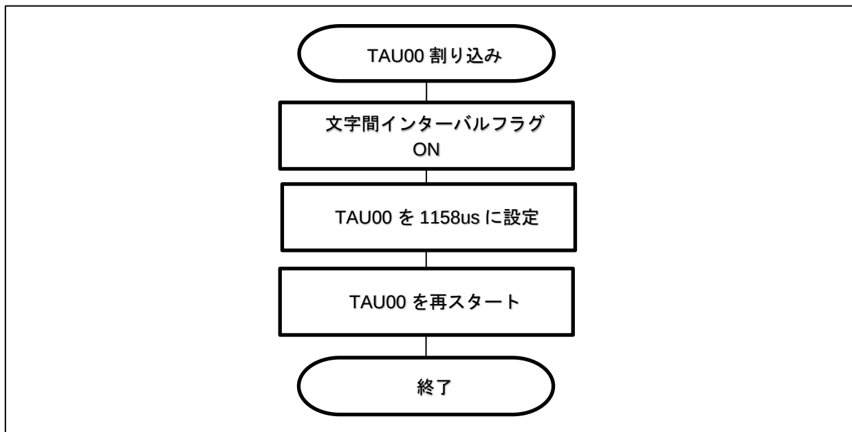
図 5-16 文字間インターバル割り込み処理（マスタモード（RTU））
