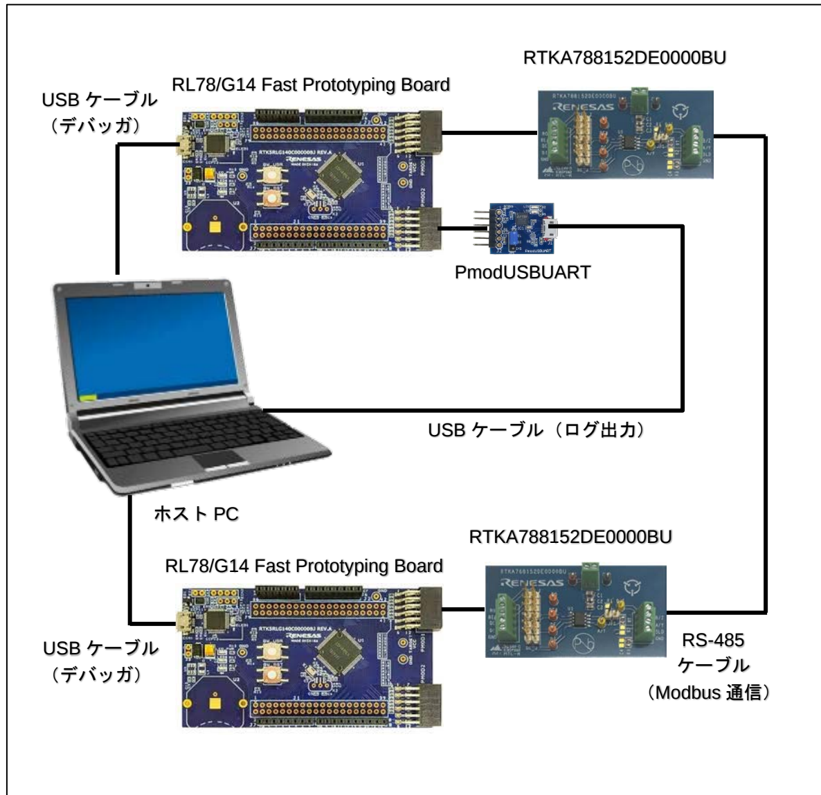
図 4-2 RL78 – RL78 環境の構成例
