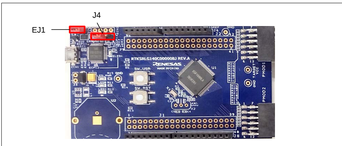
図 4-5 RL78/G14 Fast Prototyping Board ジャンパピン接続写真
