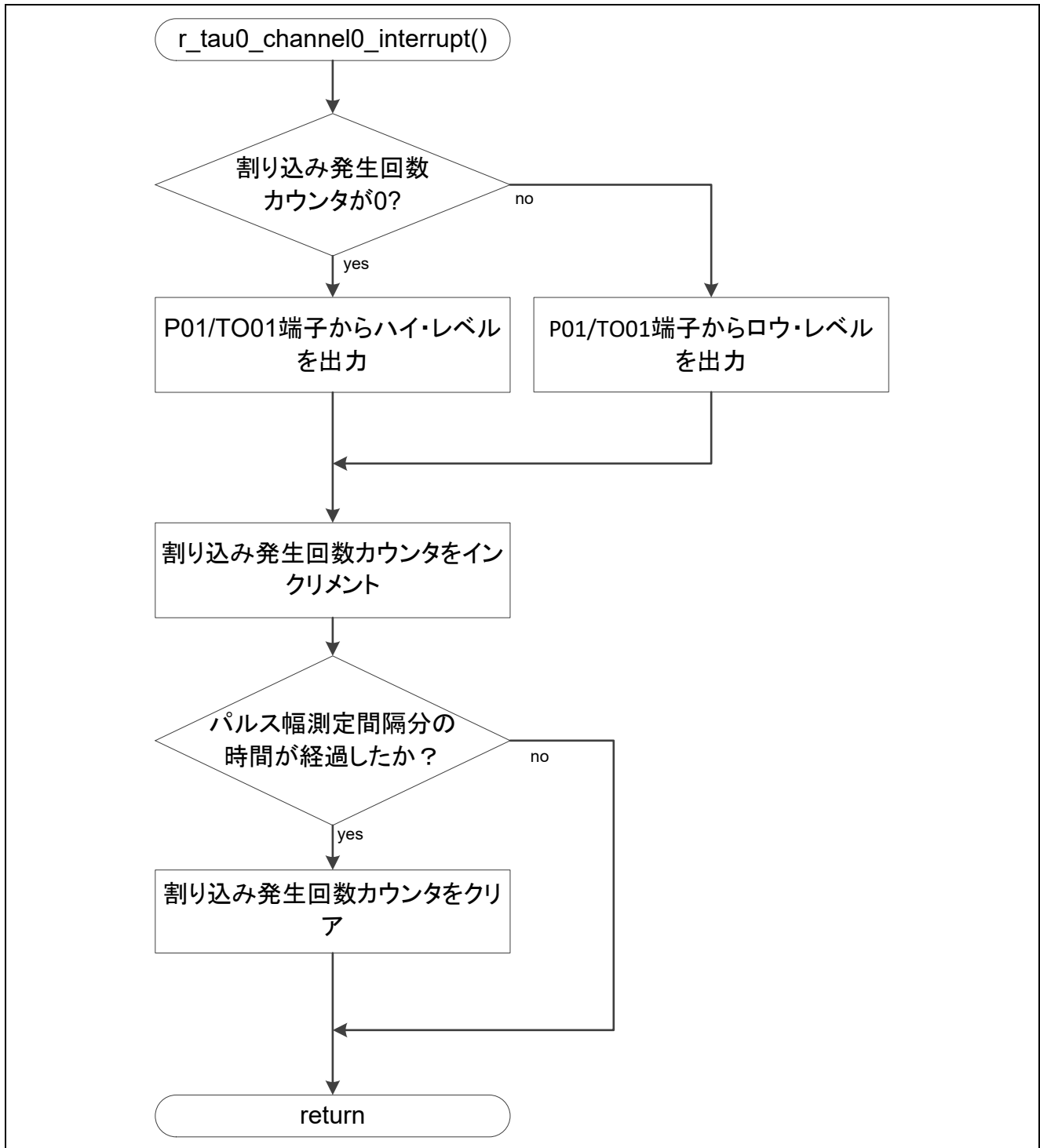
図 5.19 TAU00 割り込み関数
