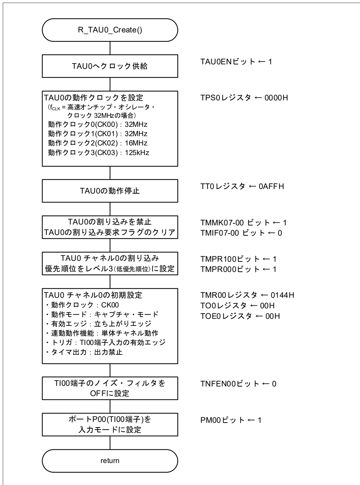
図 5.6 タイマ・アレイ・ユニット 0 の設定
