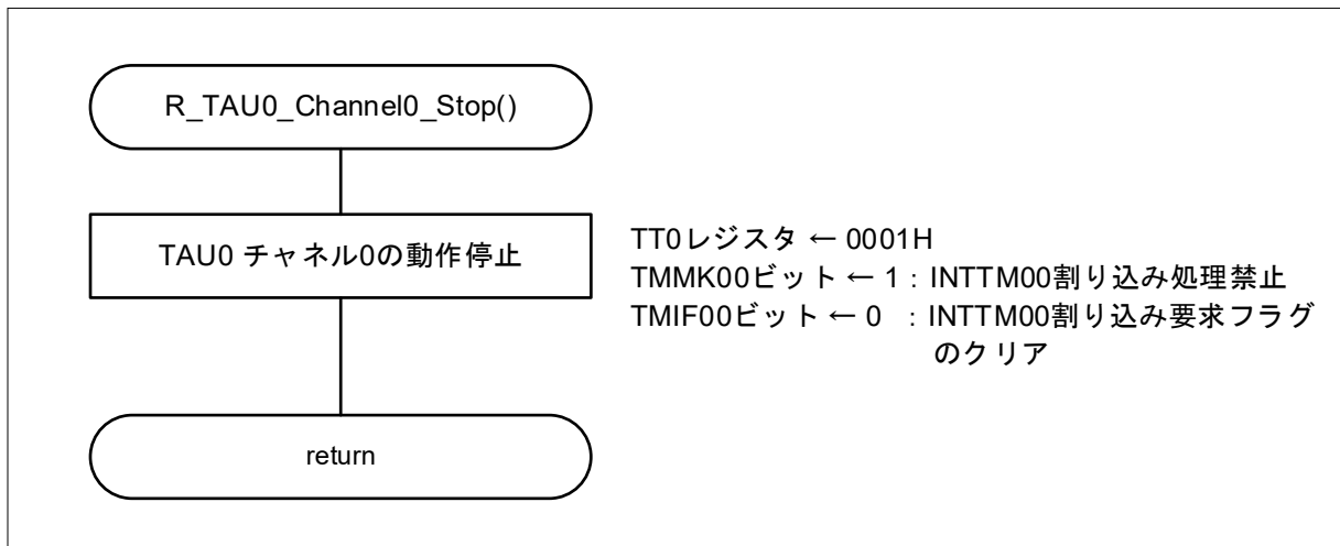
図 5.11 タイマ・アレイ・ユニット0チャンネル0動作停止
