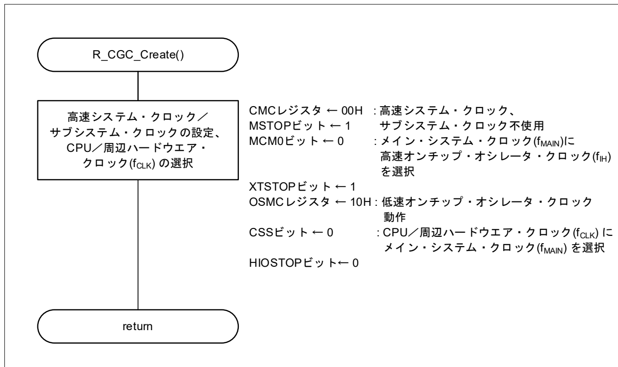
図 5.5 CPU クロックの設定
