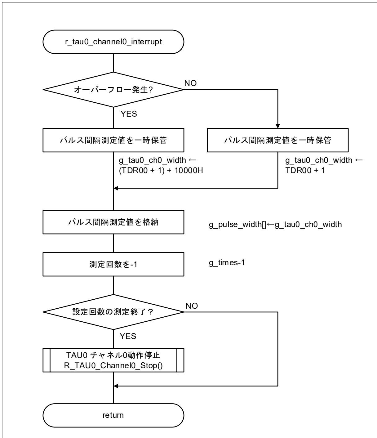
図 5.10 INTTM00 割り込み処理
