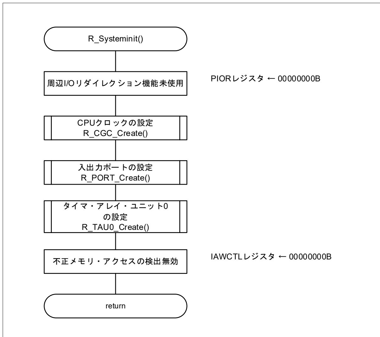
図 5.3 システム関数
