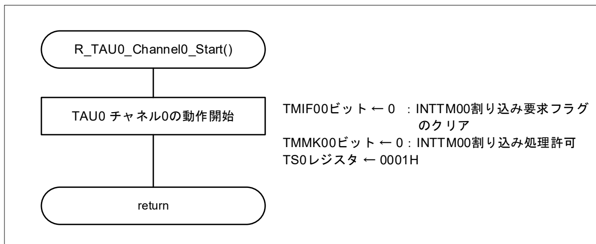
図 5.9 タイマ・アレイ・ユニット 0 チャンネル 0 動作開始
