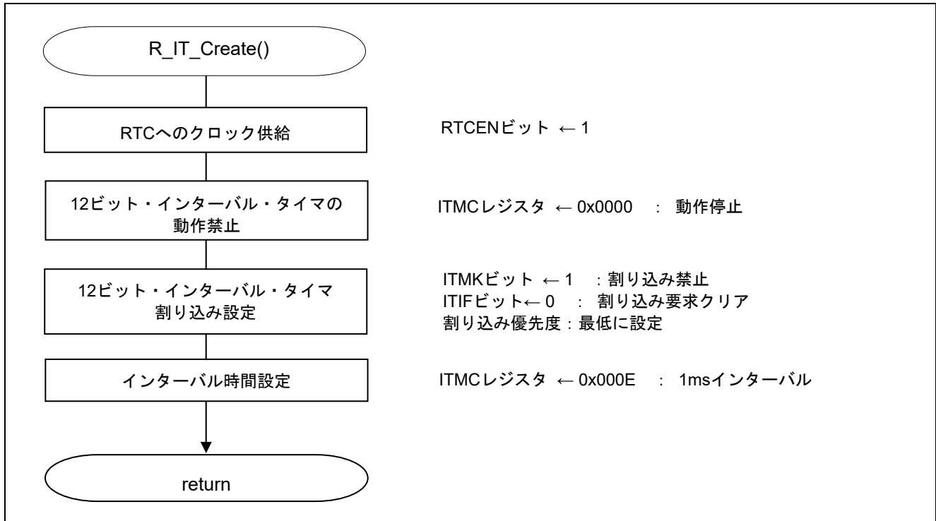
図 5.8 12 ビット・インターバル・タイマの設定
