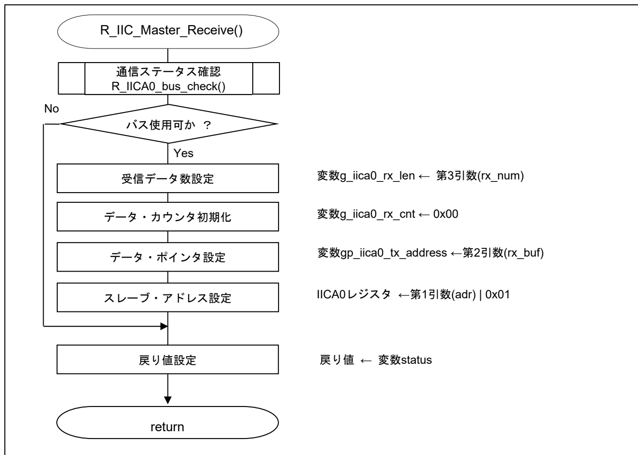
図 5.21 IICA0 マスタ受信起動関数
