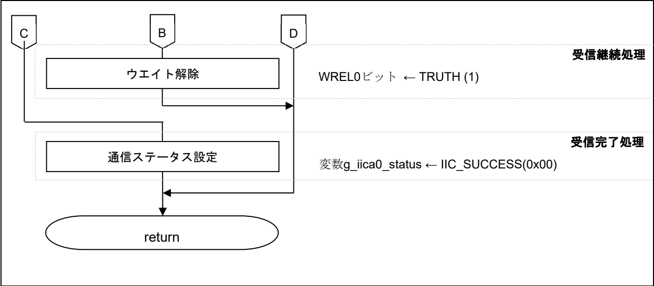
図 5.28 IICA0 割り込み処理 (3/3)
