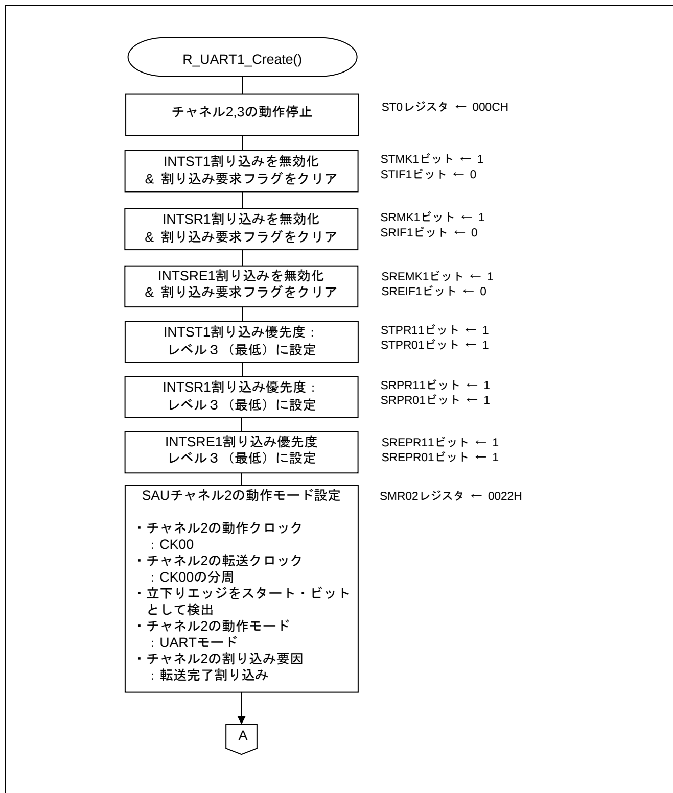
図 5.7 UART1 の設定（1/3）
