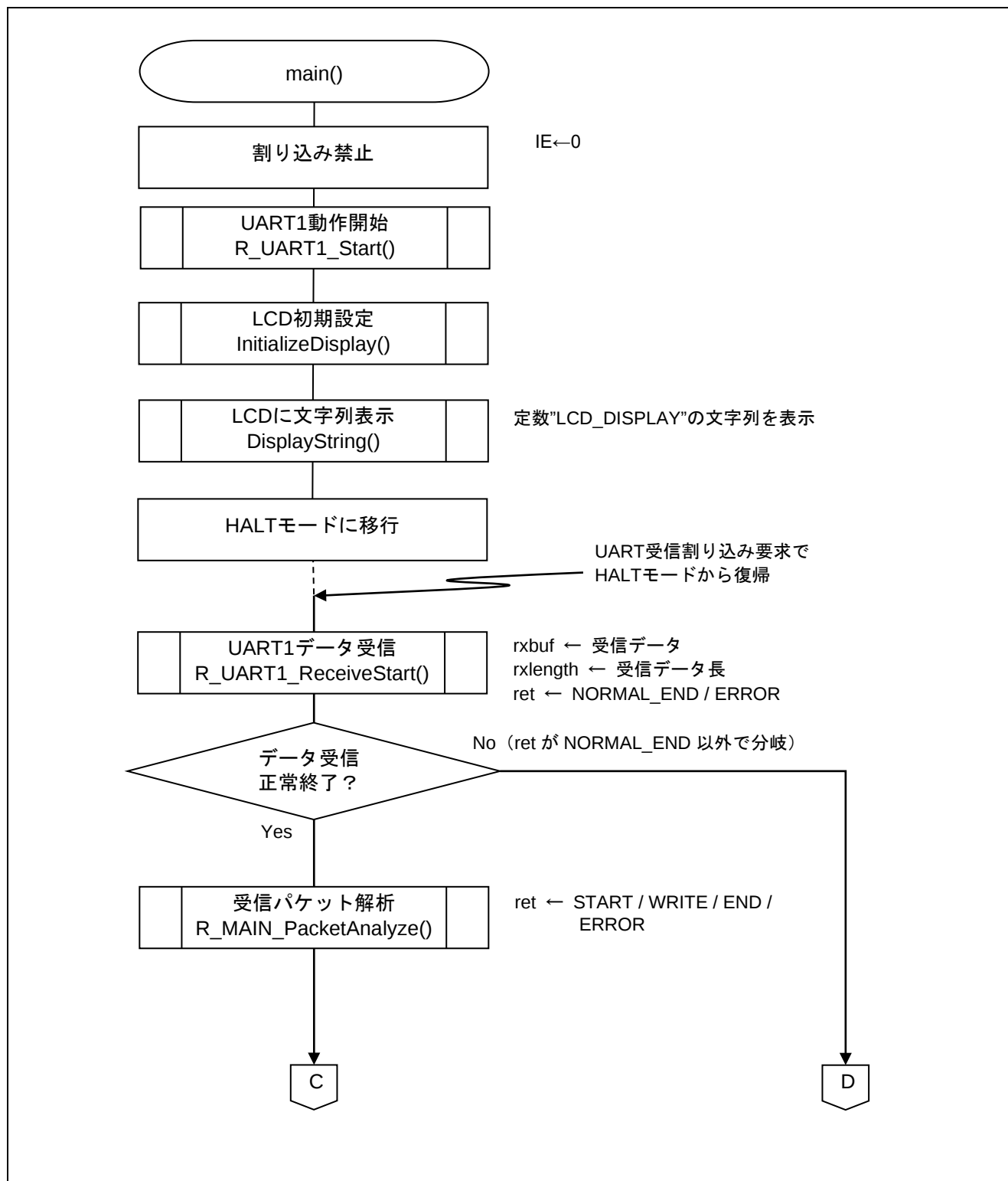
図 5.10 メイン処理(1/2)
