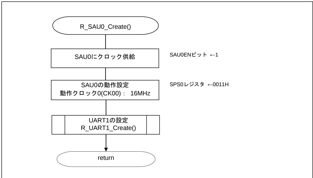
図 5.6 SAU0 の設定
