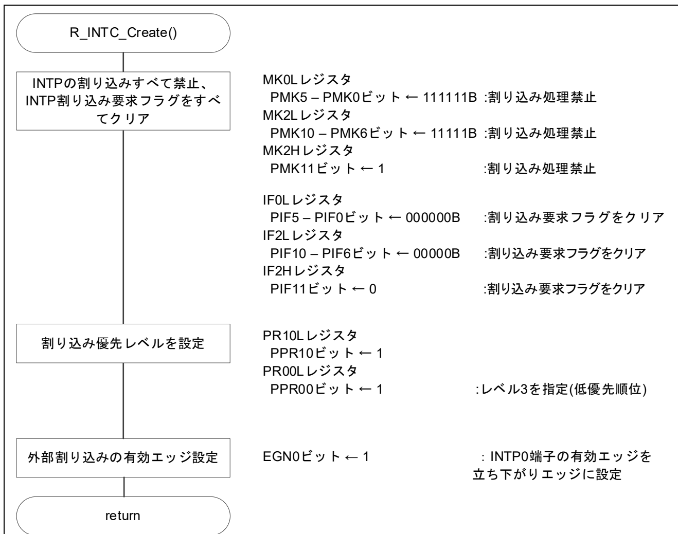
図 5.8 外部割り込み初期設定関数
