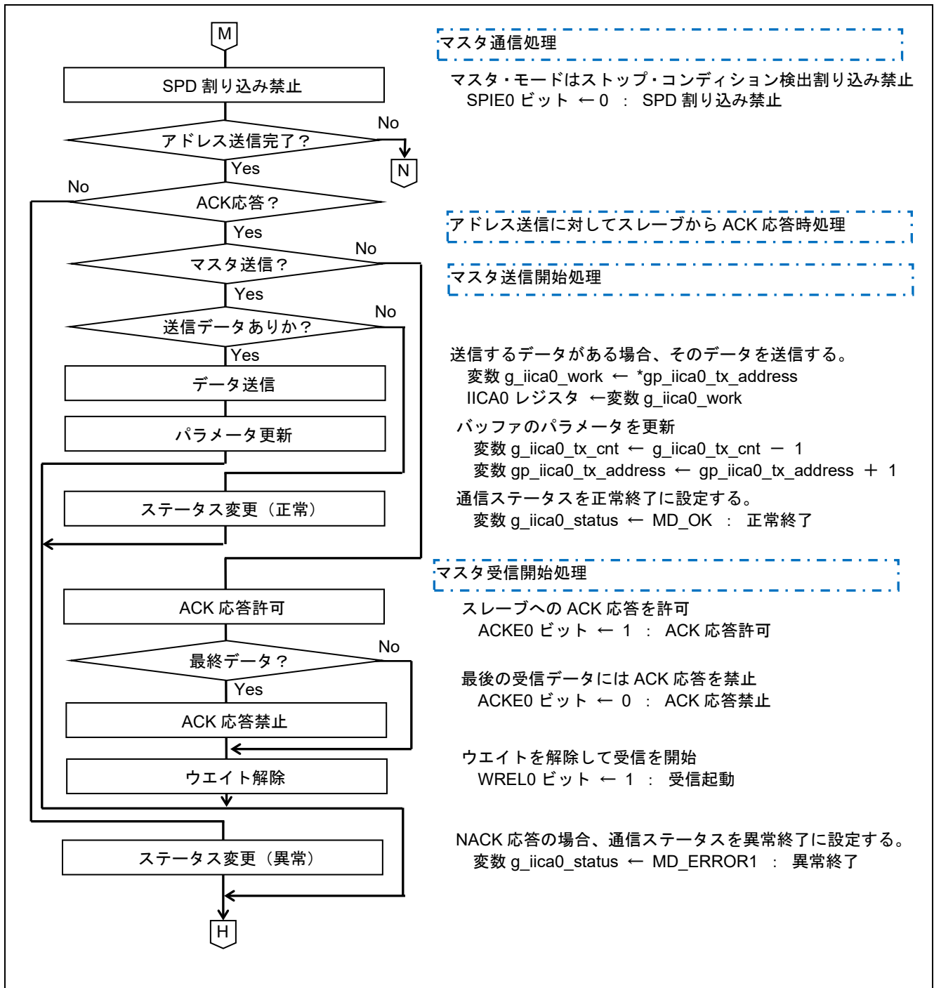
図 5.23 IICA0 割り込み処理 (4/5)
