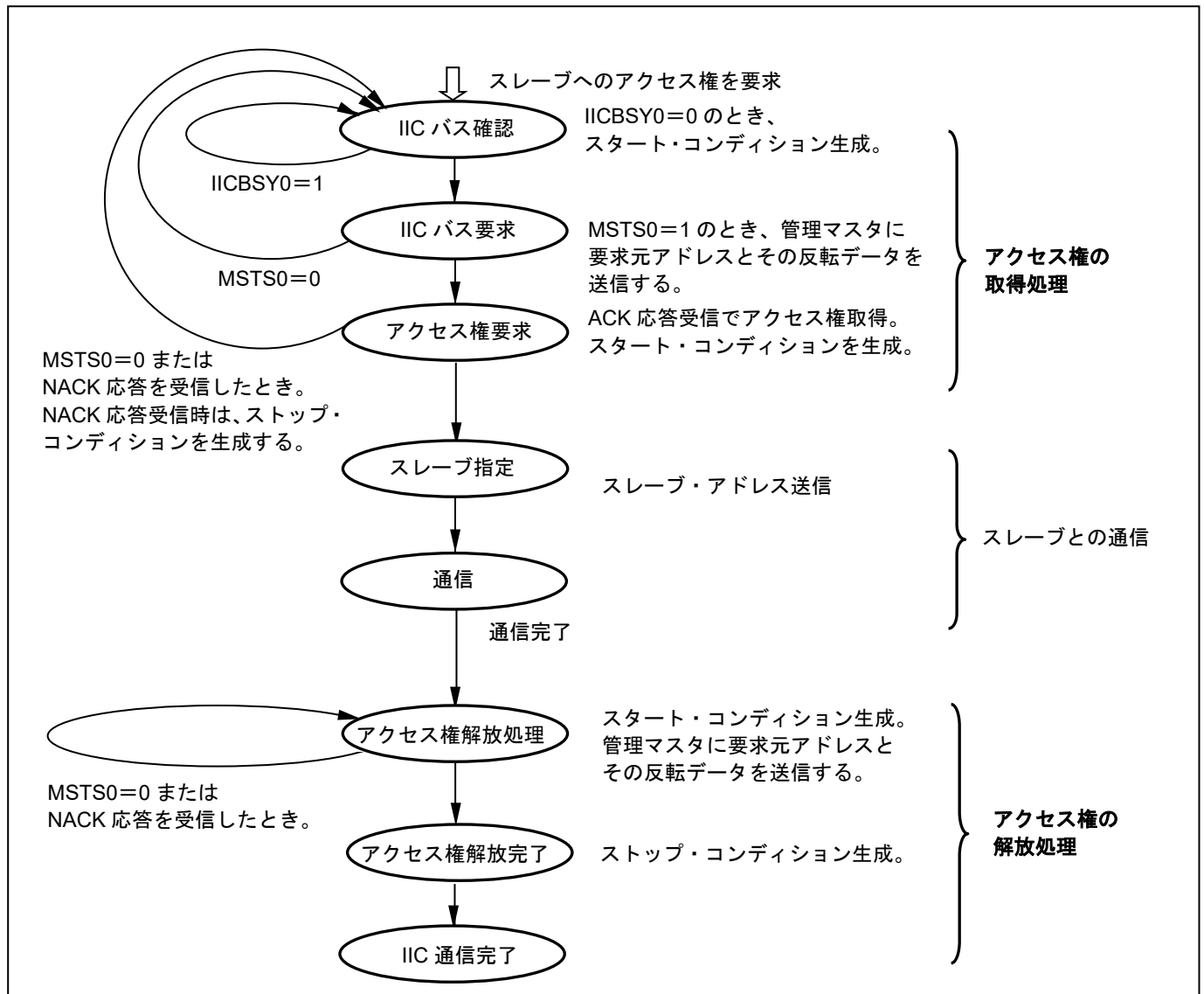
図 1.7 クライアント処理（概略）
