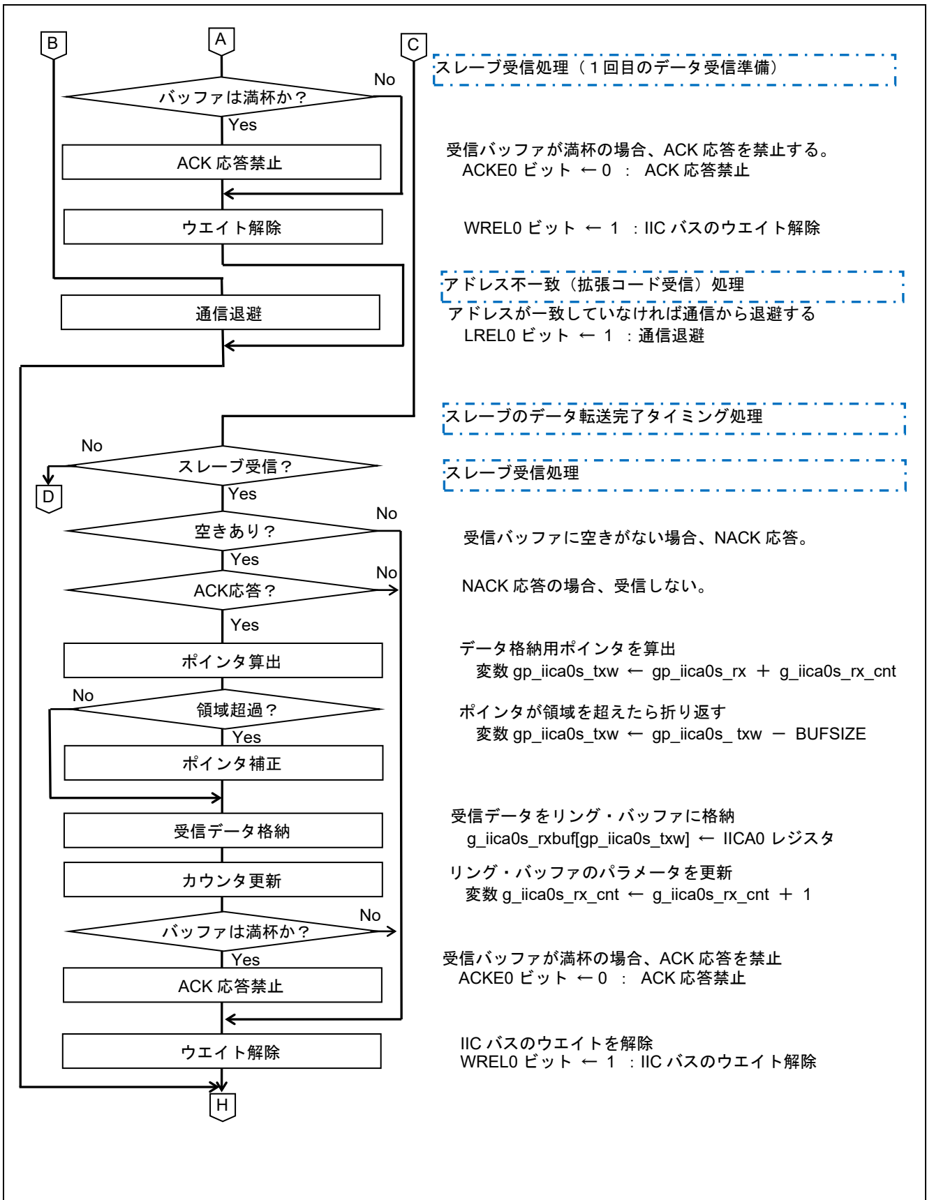
図 5.21 IICA0 割り込み処理 (2/5)
