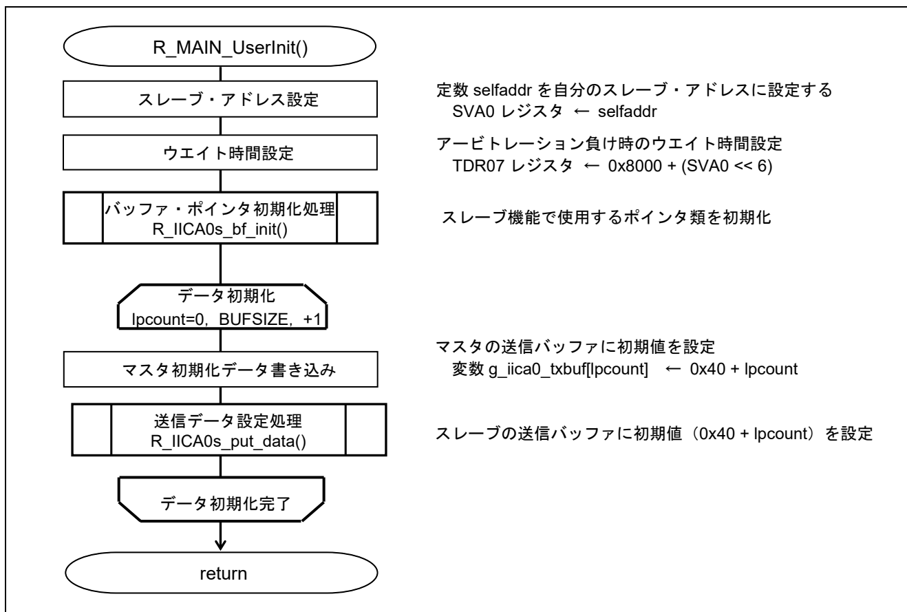
図 5.10 システムの初期化処理関数
