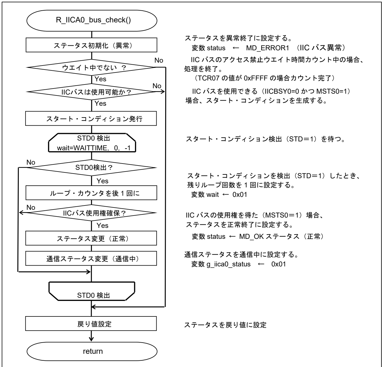
図 5.18 IIC バス状態確認／スタート・コンディション生成処理
