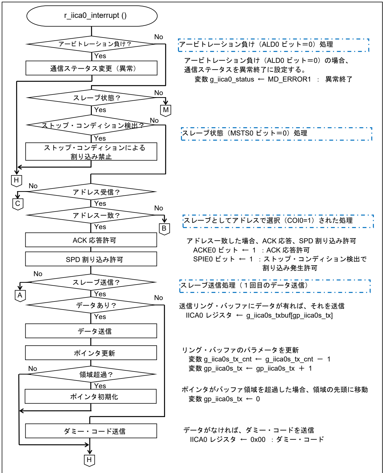
図 5.20 IICA0 割り込み処理 (1/5)
