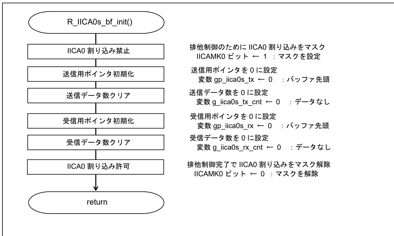
図 5.15 バッファ・ポインタ初期化処理
