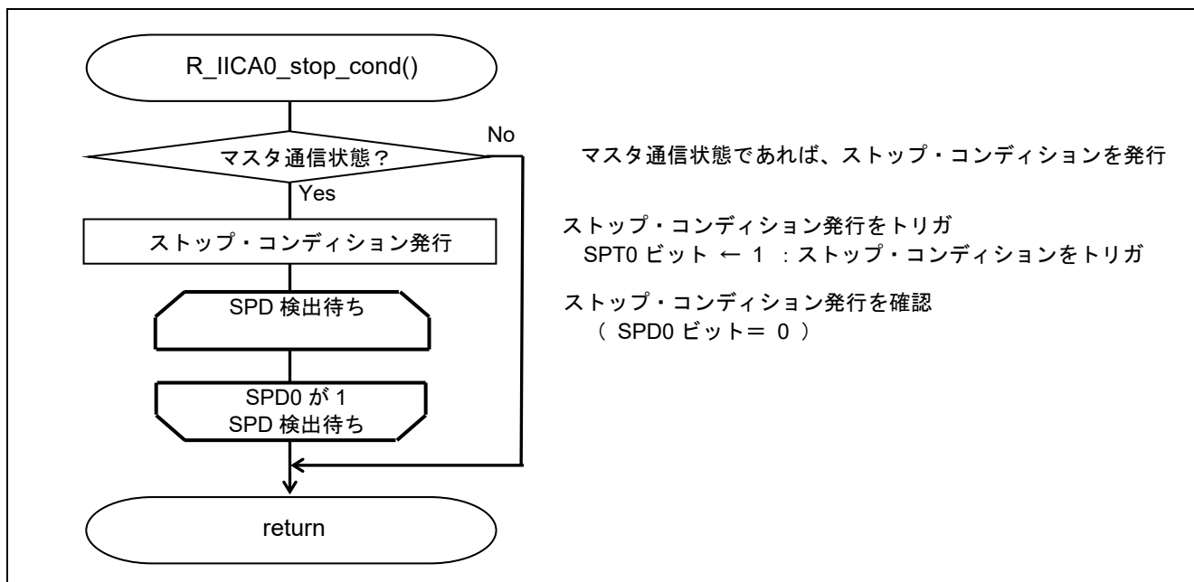
図 5.19 ストップ・コンディション生成処理
