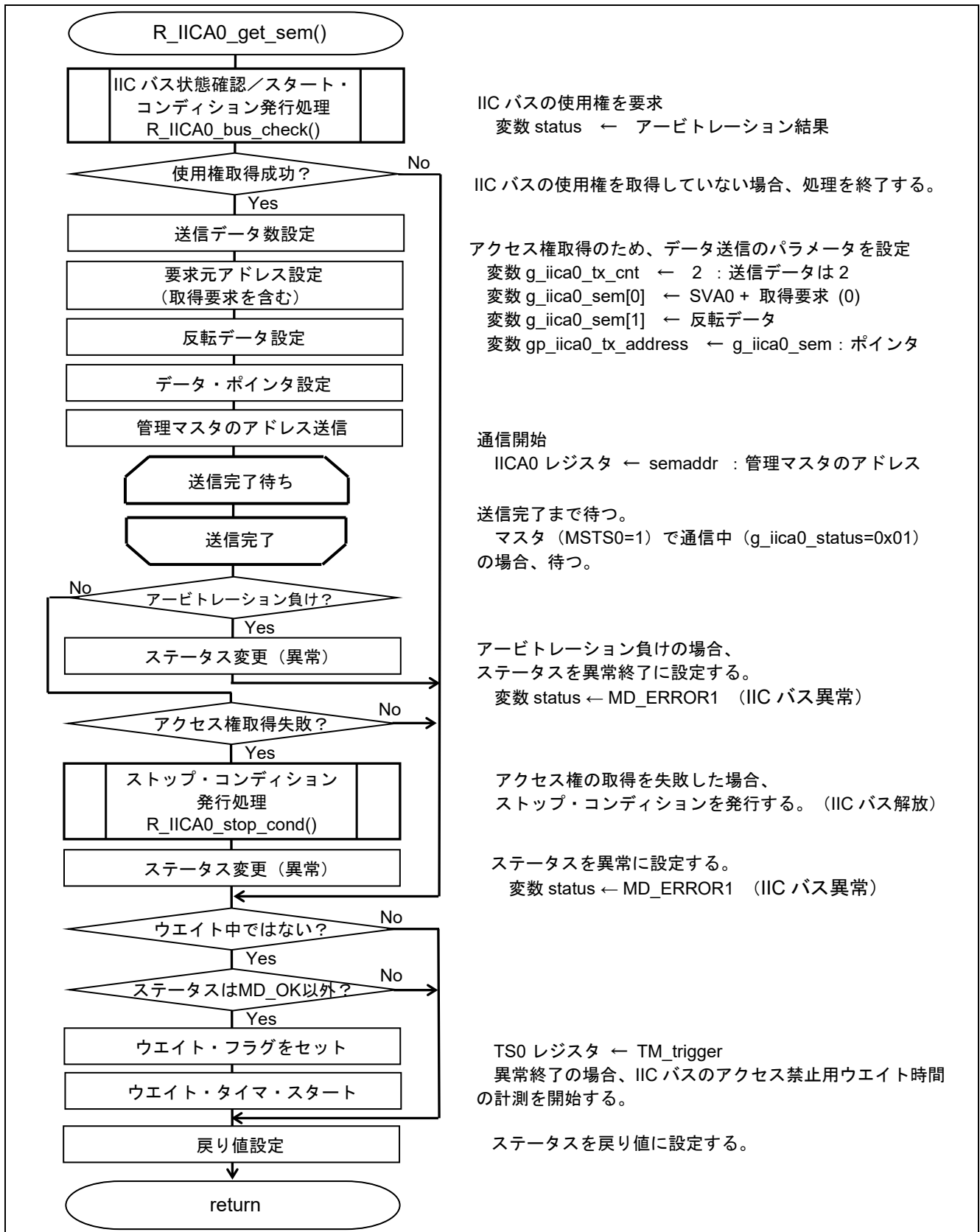
図 5.17 アクセス権取得処理
