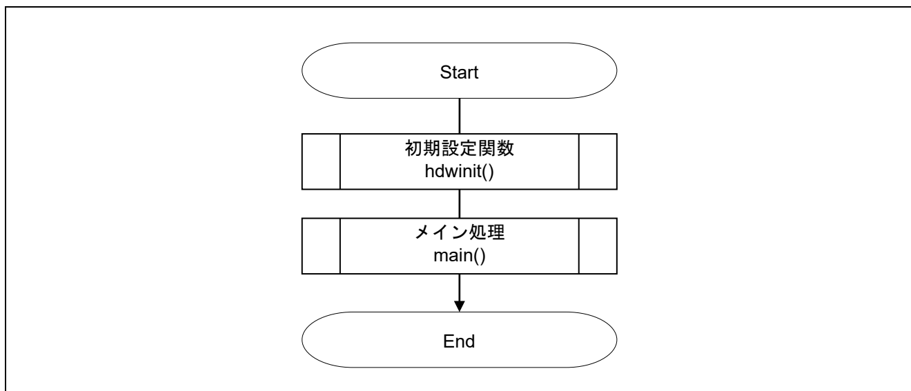
図 5.1 全体フロー
