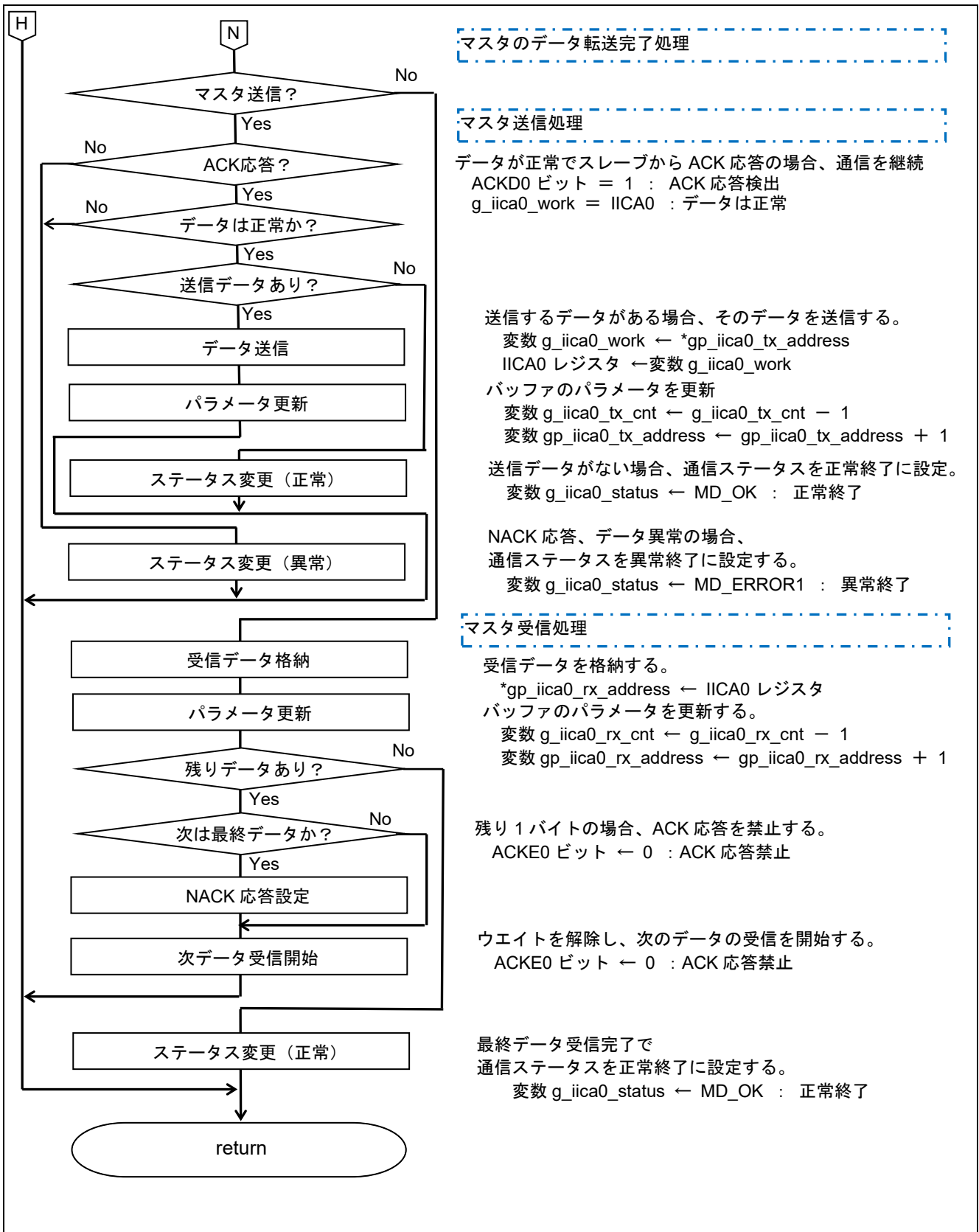
図 5.24 IICA0 割り込み処理 (5/5)
