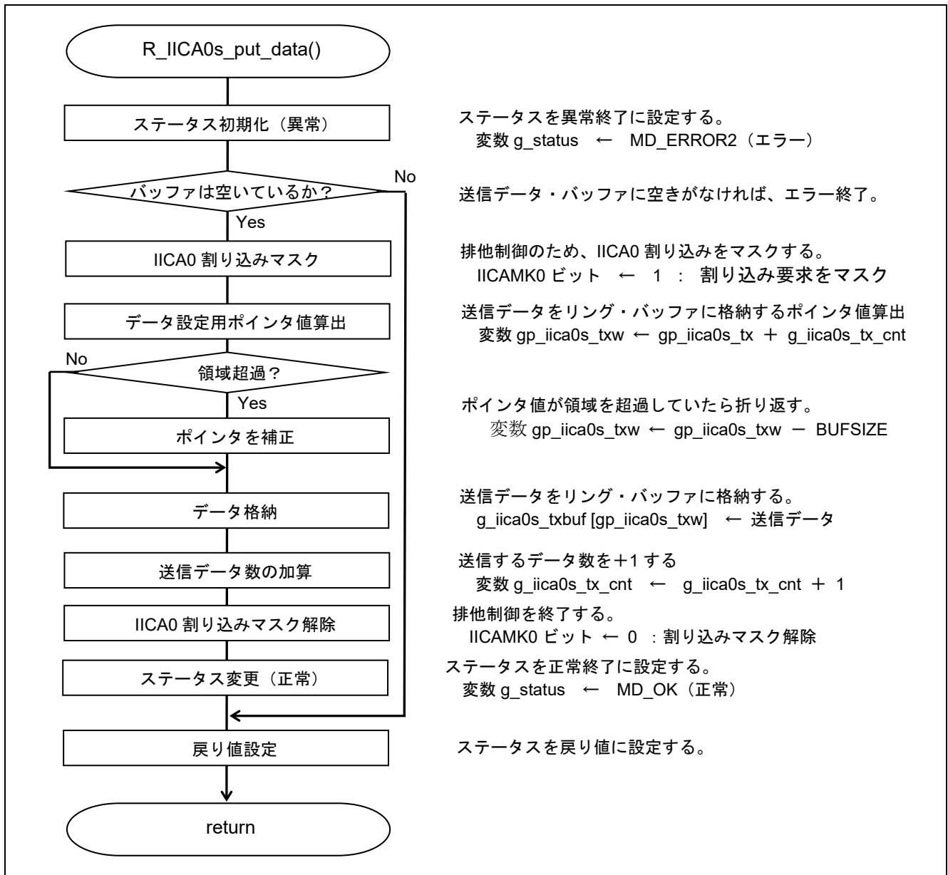
図 5.16 スレーブ送信データ追加処理
