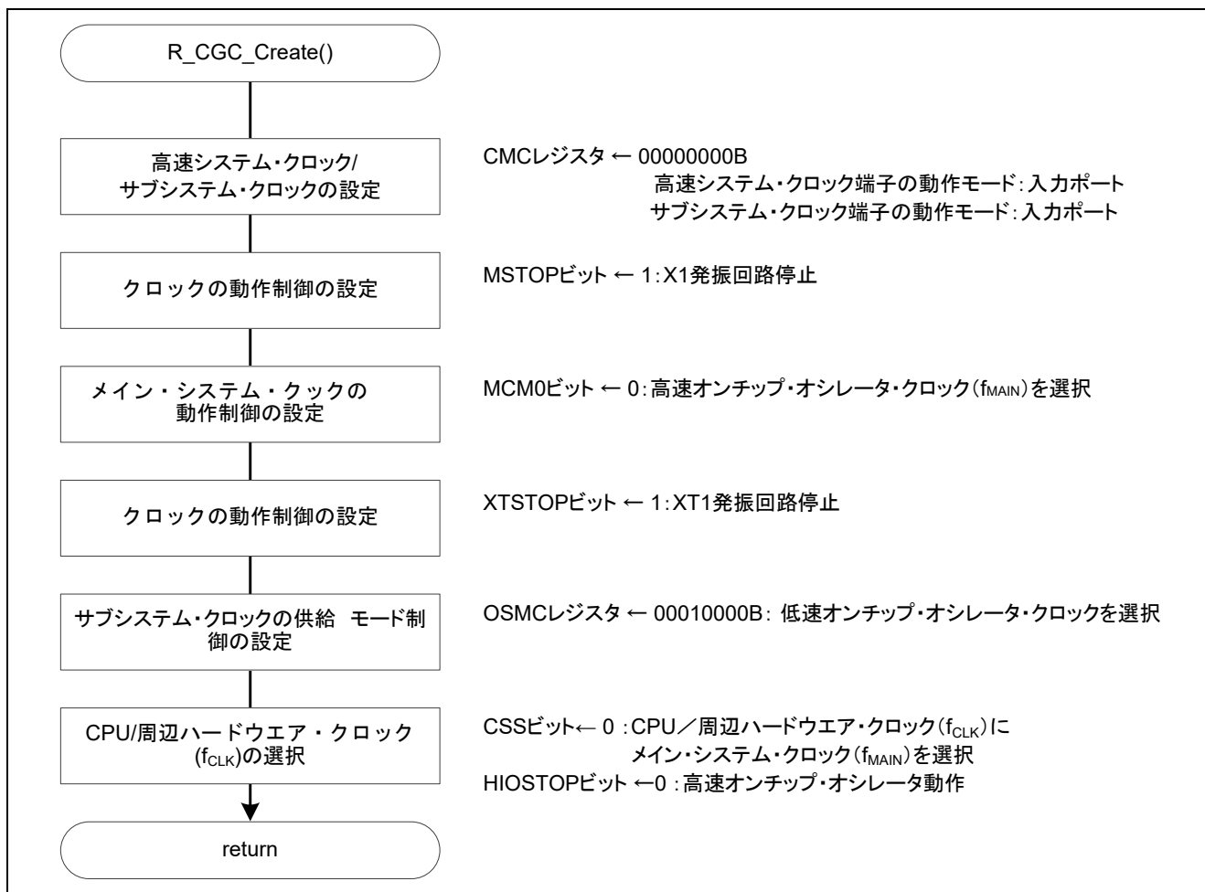
図 5.4 CPU クロック初期設定関数
