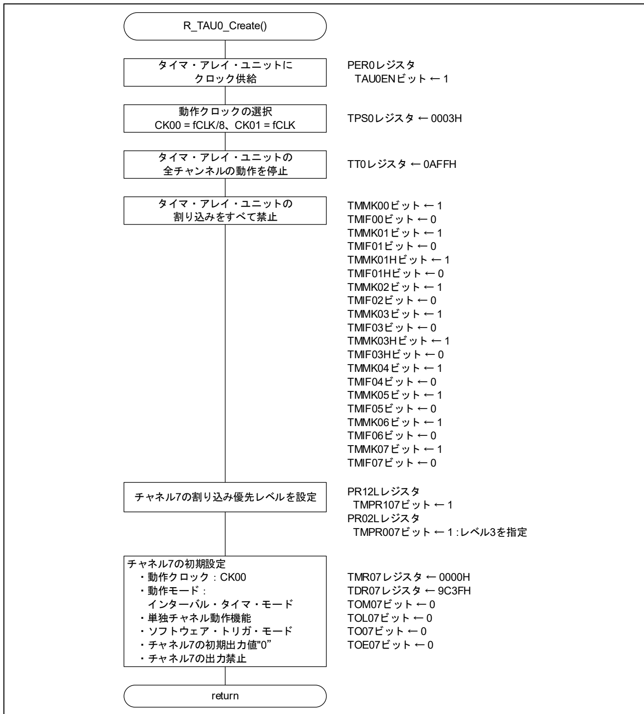
図 5.7 タイマ・アレイ・ユニット初期設定関数
