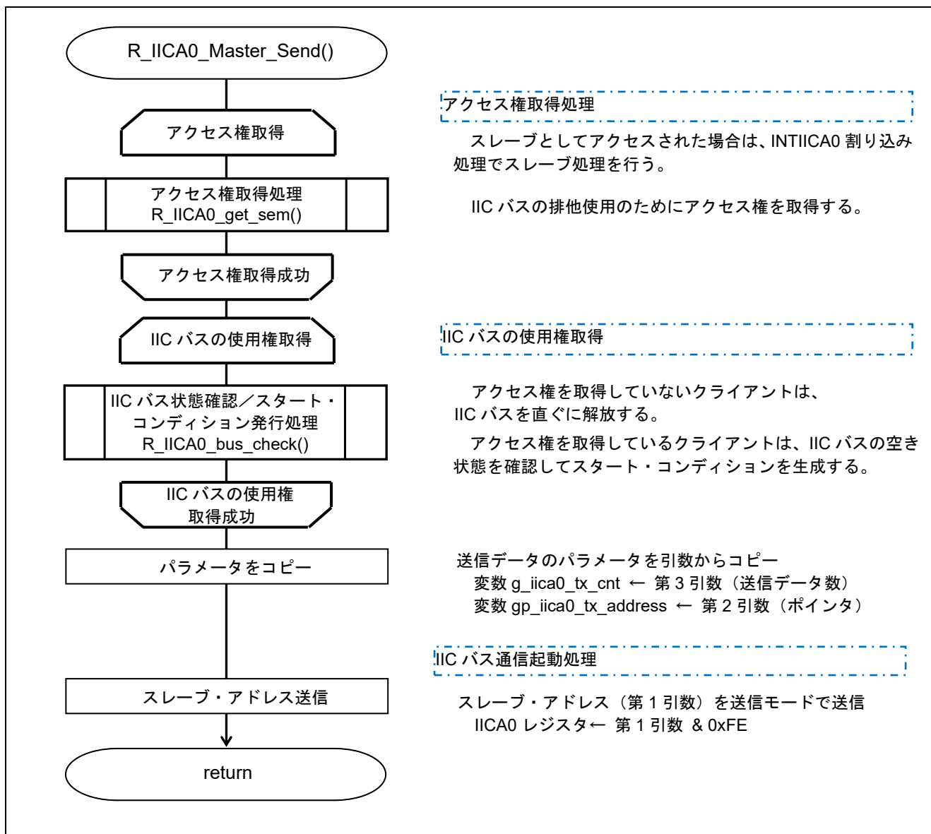
図 5.11 マスタ送信起動処理
