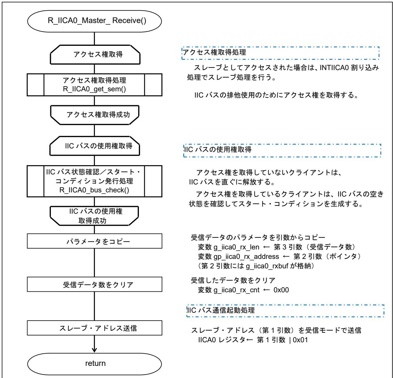
図 5.13 マスタ受信起動処理
