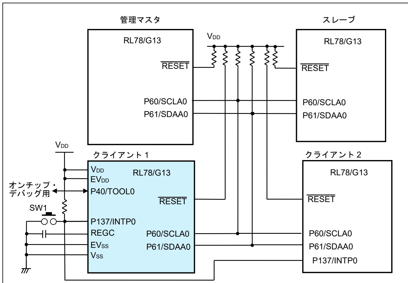
図 4.1 ハードウェア構成
