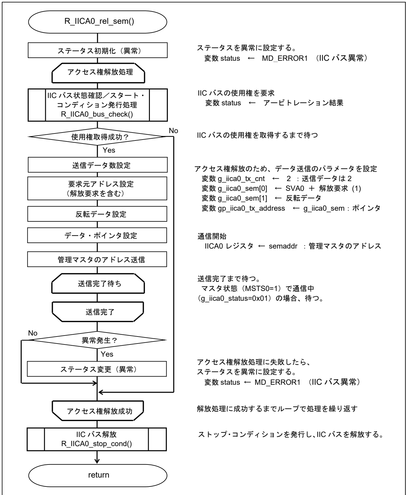
図 5.14 アクセス権解放処理
