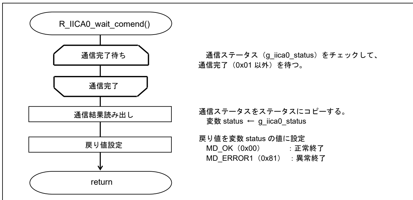
図 5.12 通信完了待ち処理関数
