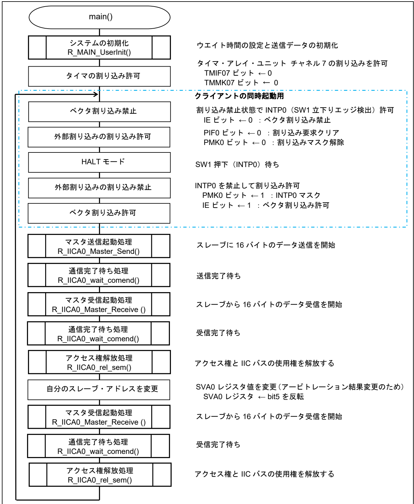
図 5.9 メイン関数
