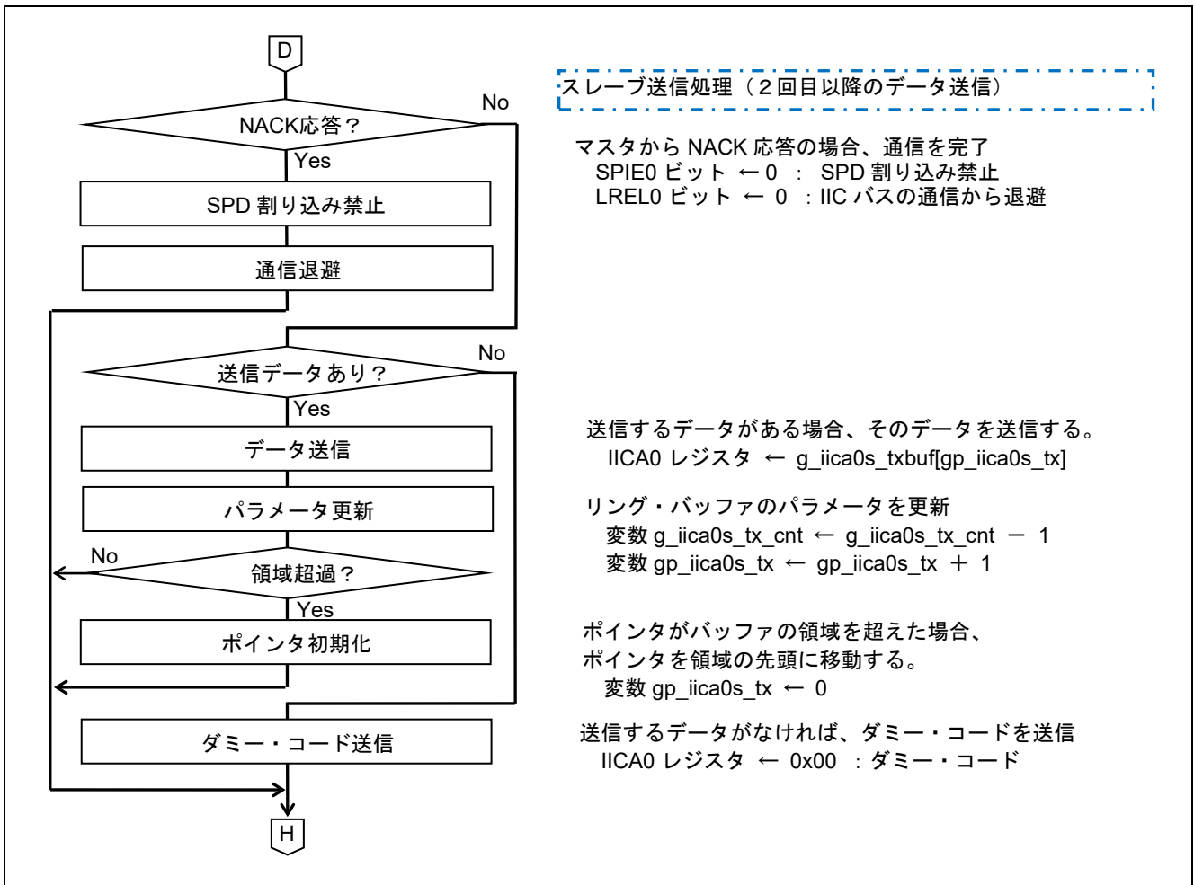
図 5.22 IICA0 割り込み処理 (3/5)
