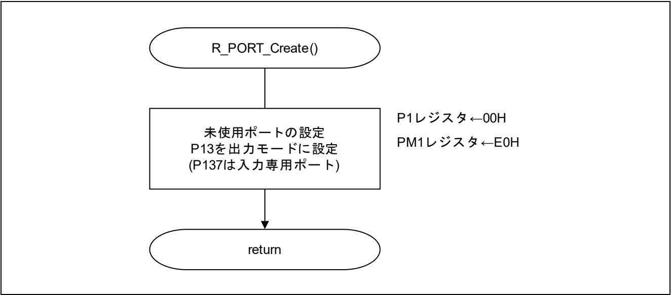
図 5.4 入出力ポートの設定
