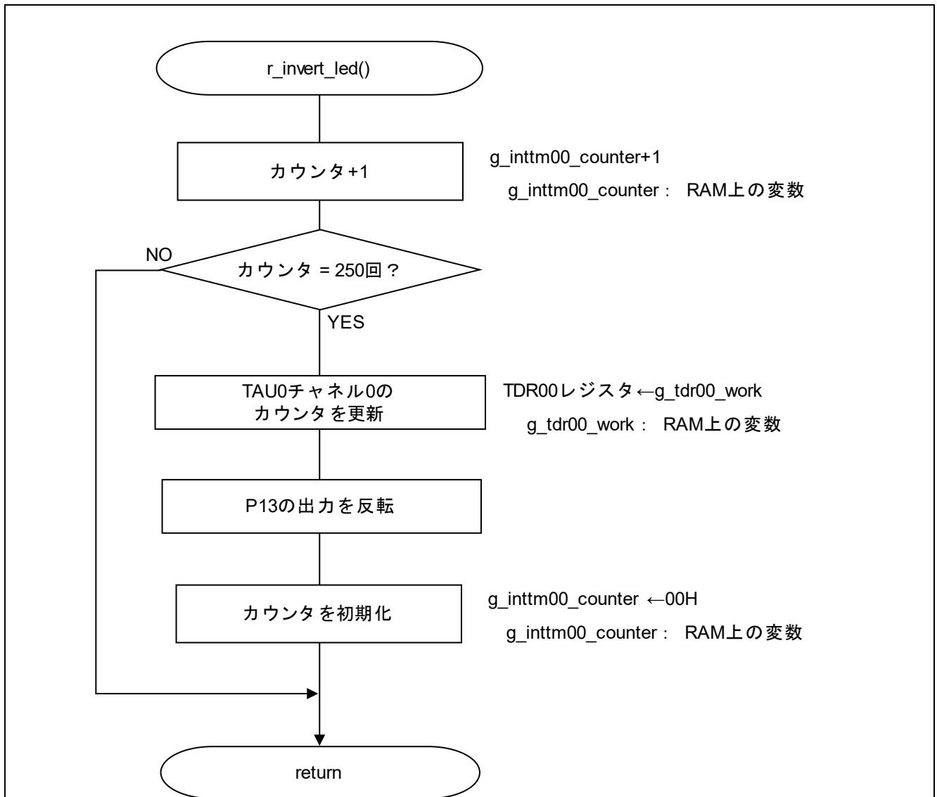
図 5.13 666ms 経過判定処理
