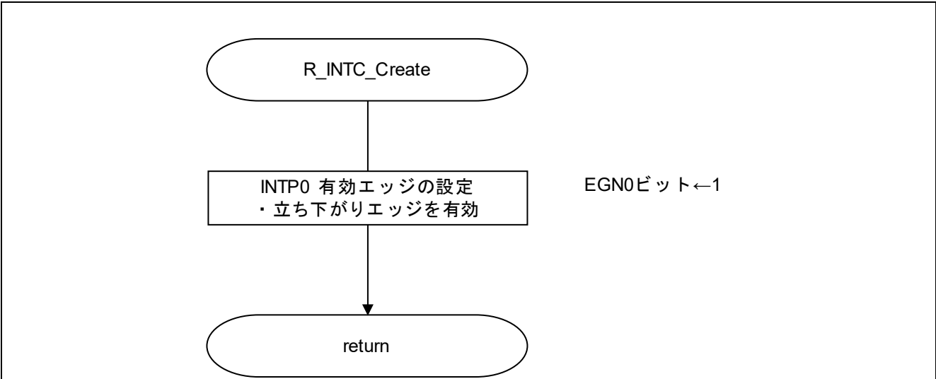
図 5.7 INTC モジュールの設定
