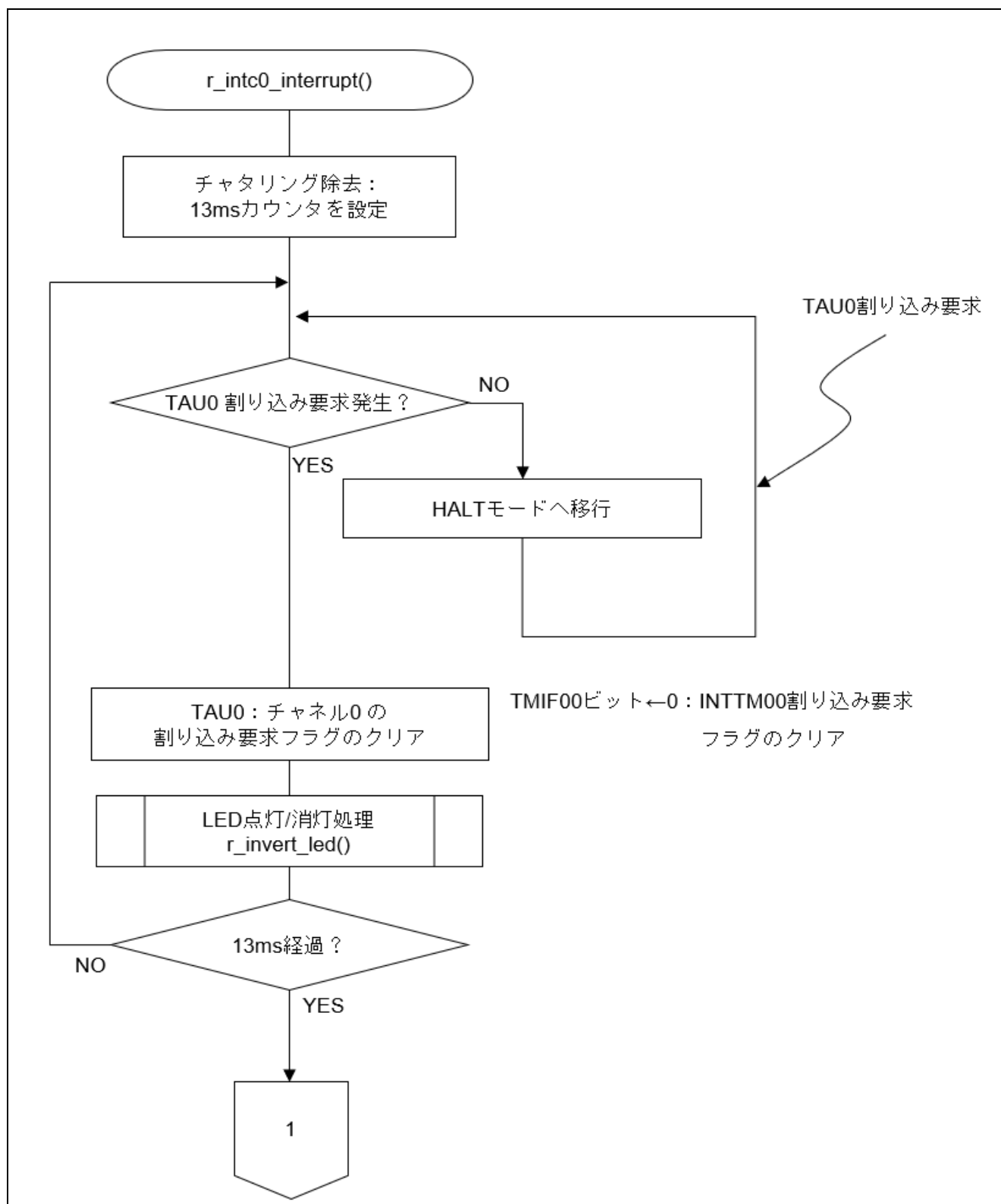
図 5.14 INTP0 割り込み処理 (1/2)
