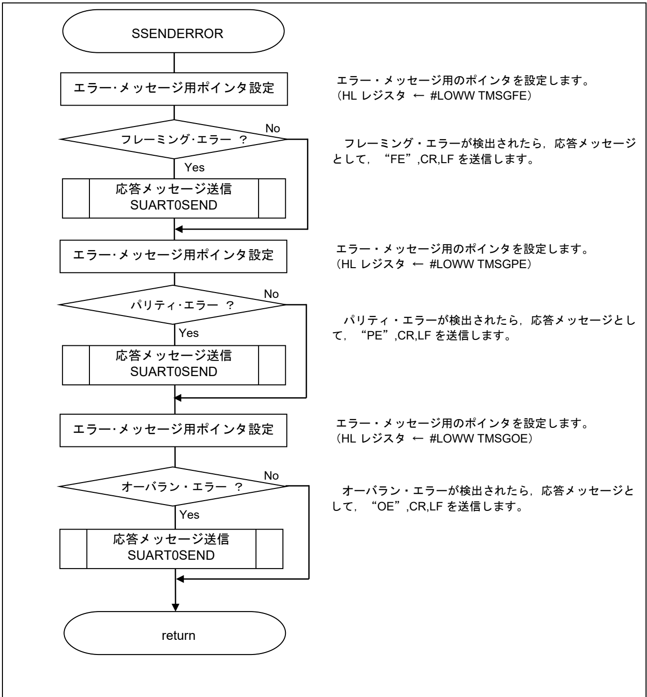
図 5.8 エラー応答メッセージ送信処理関数
