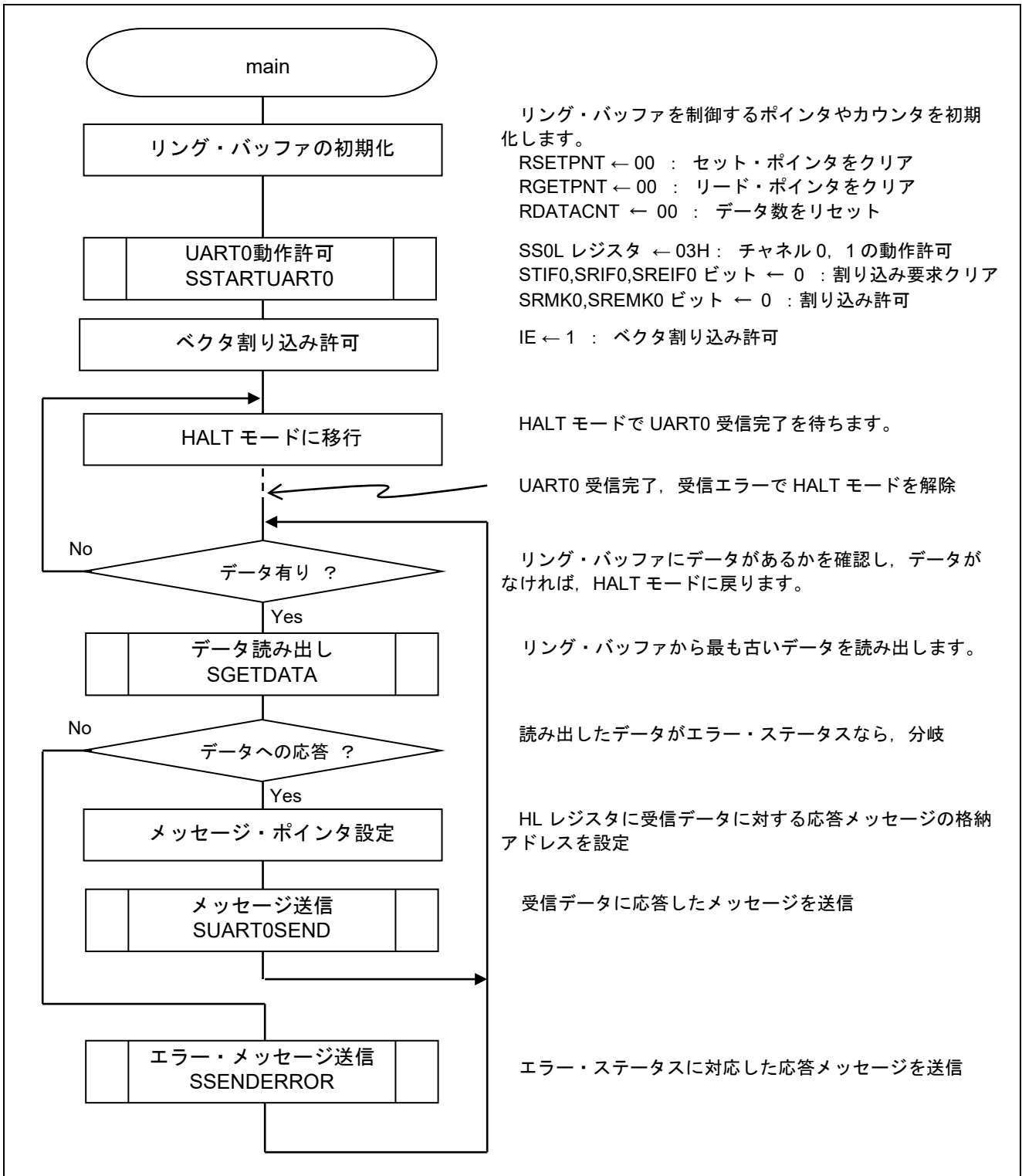
図 5.6 メイン処理
