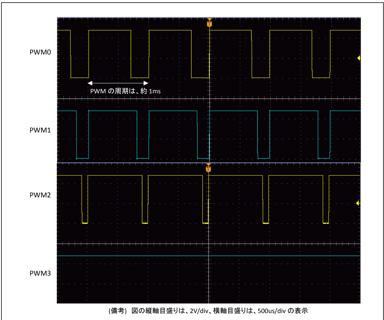
図 6.3 外部スイッチ押下 2 回目の多重 PWM 出力波形
