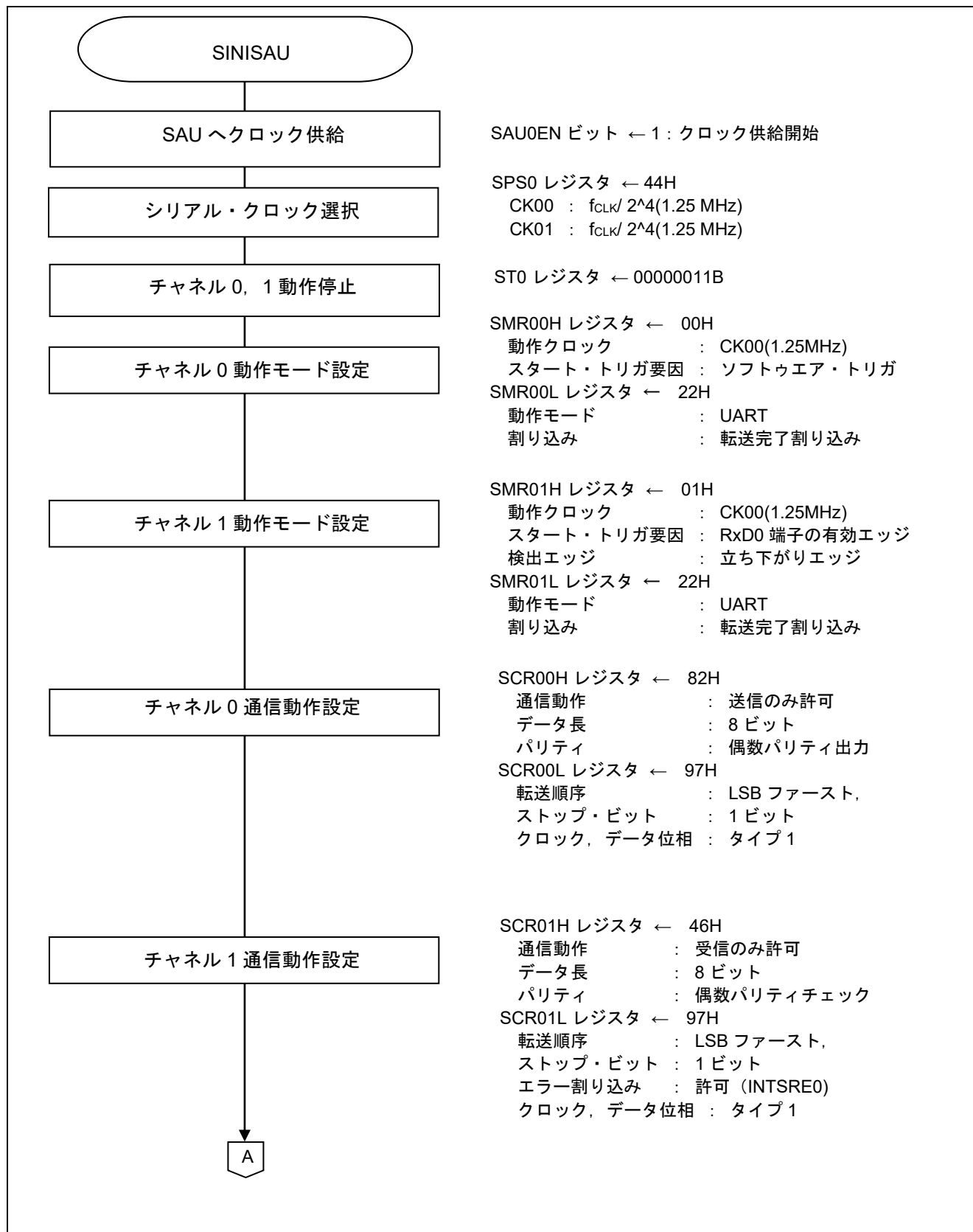
図 5.5 SAU の設定 (1/2)
