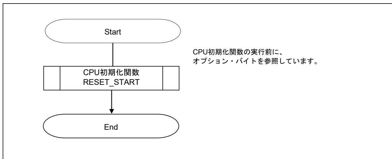
図 5.1 全体フロー
