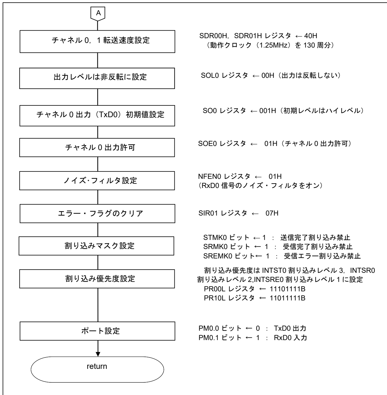
図 5.6 SAU の設定 (2/2)
