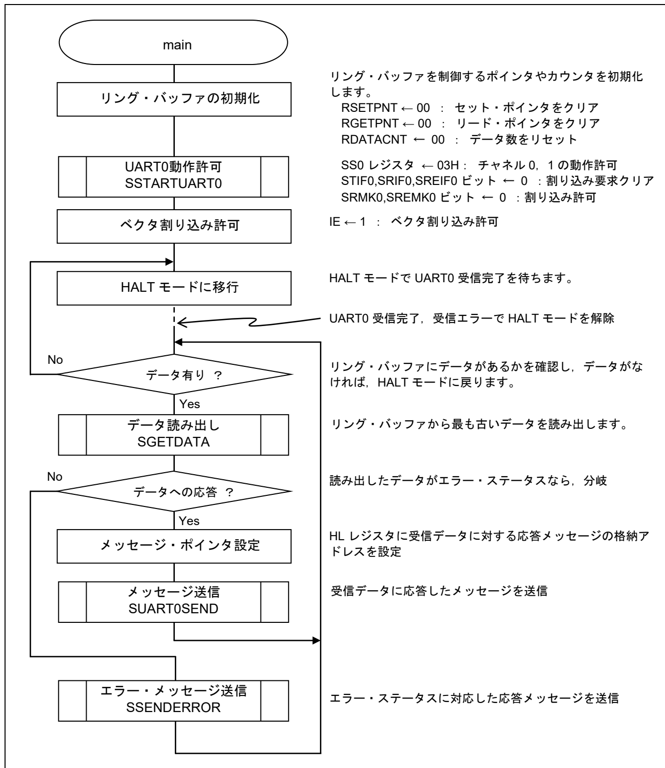
図 5.7 メイン処理
