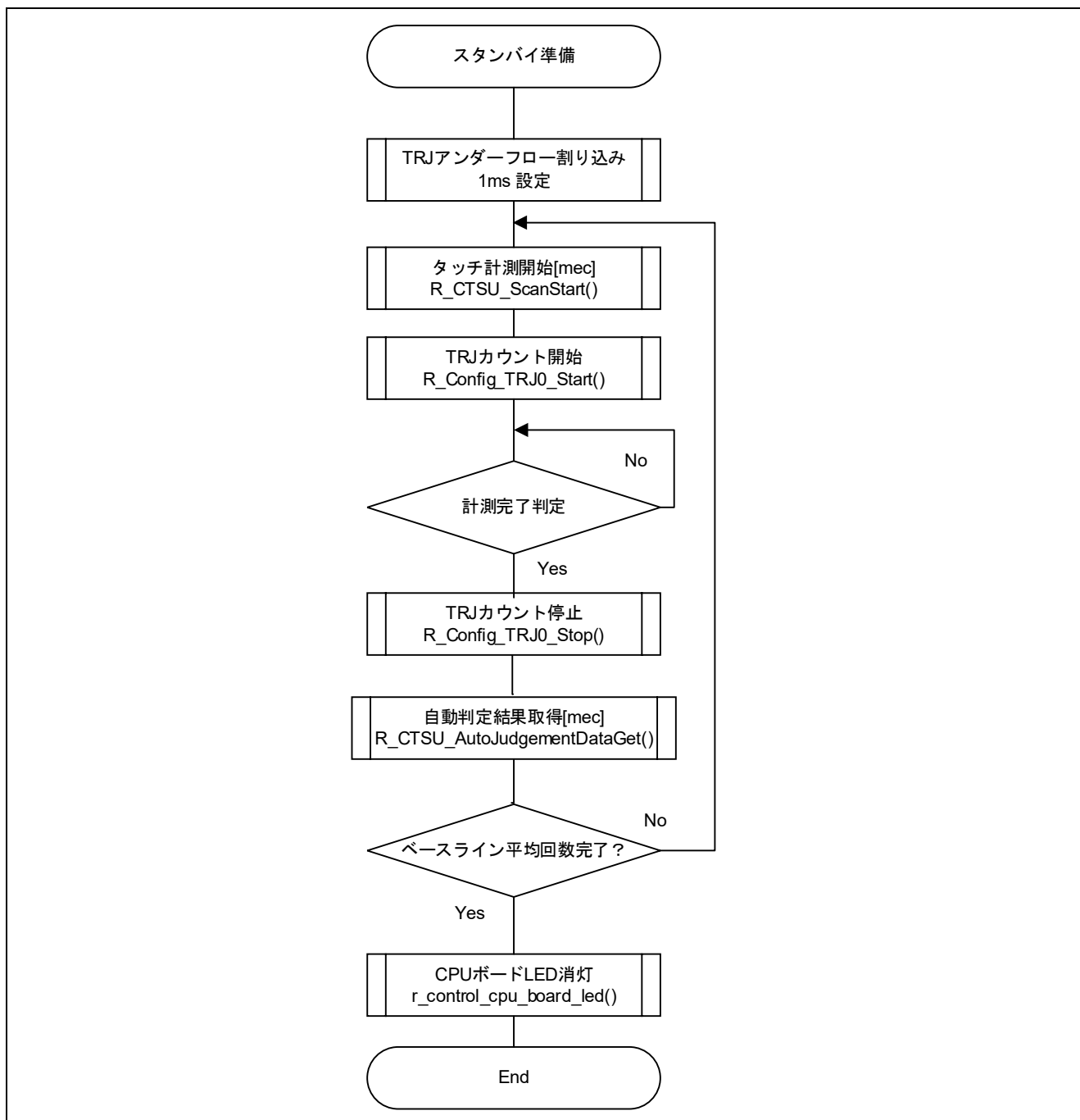
図 5.6 スタンバイ準備のフローチャート
