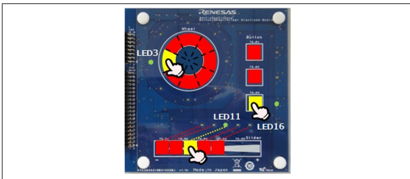
図 5.11 タッチ電極と LED の動作
