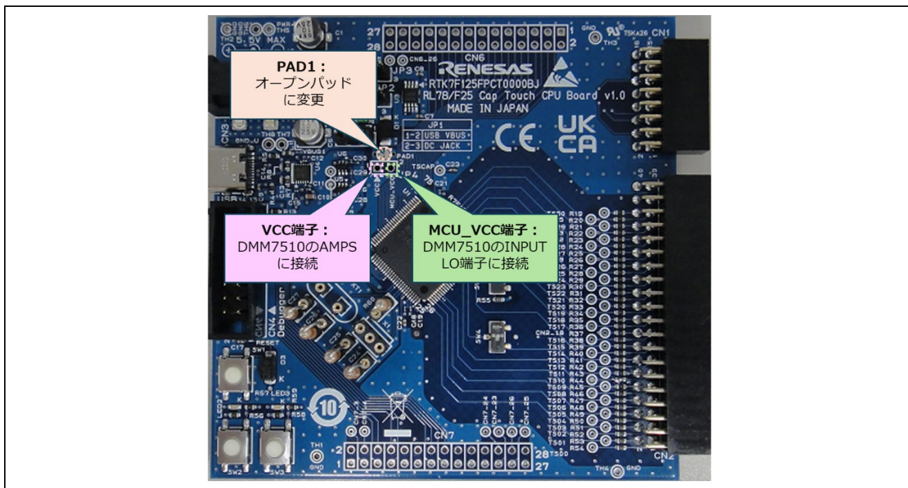
図 7.1 RL78/F25 CPU ボード・前面
