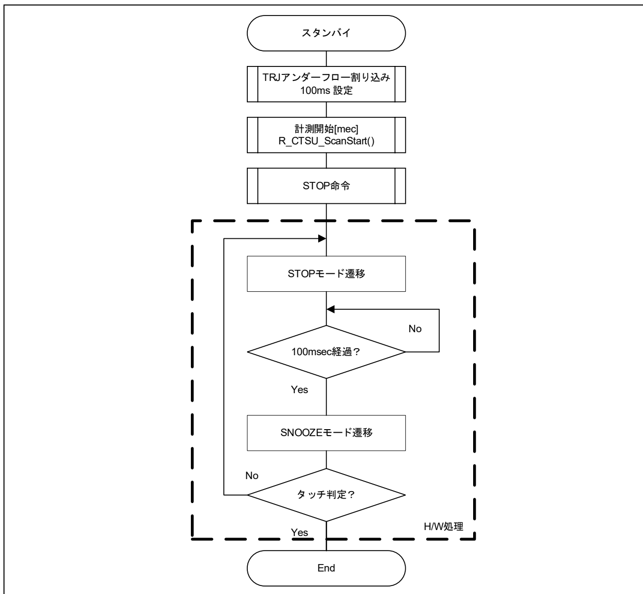
図 5.9 スタンバイのフローチャート
