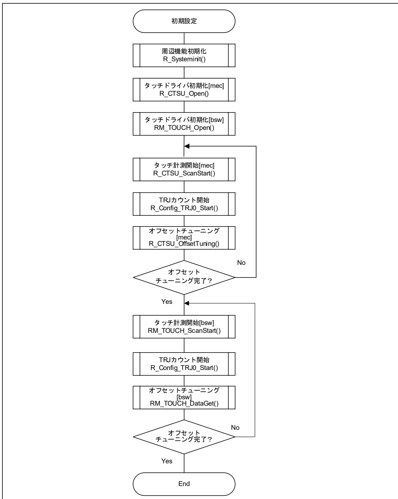
図 5.5 初期設定処理のフローチャート
