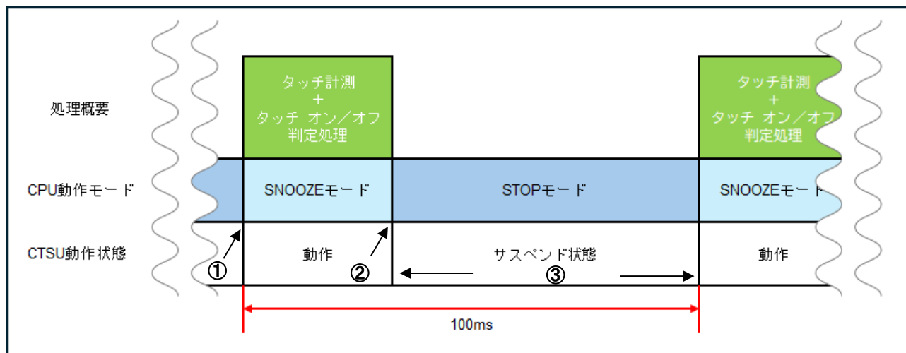
図 5.8 CPU 動作モードと CTSU 動作状態のイメージ
