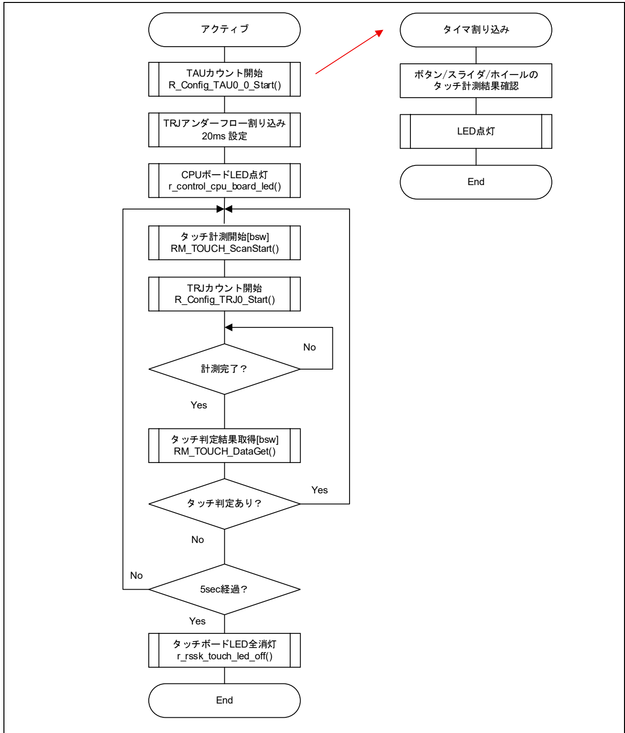
図 5.10 アクティブモードのフローチャート
