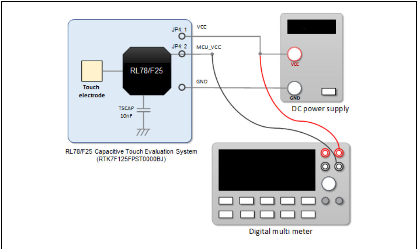
図 7.3 消費電流計測環境
