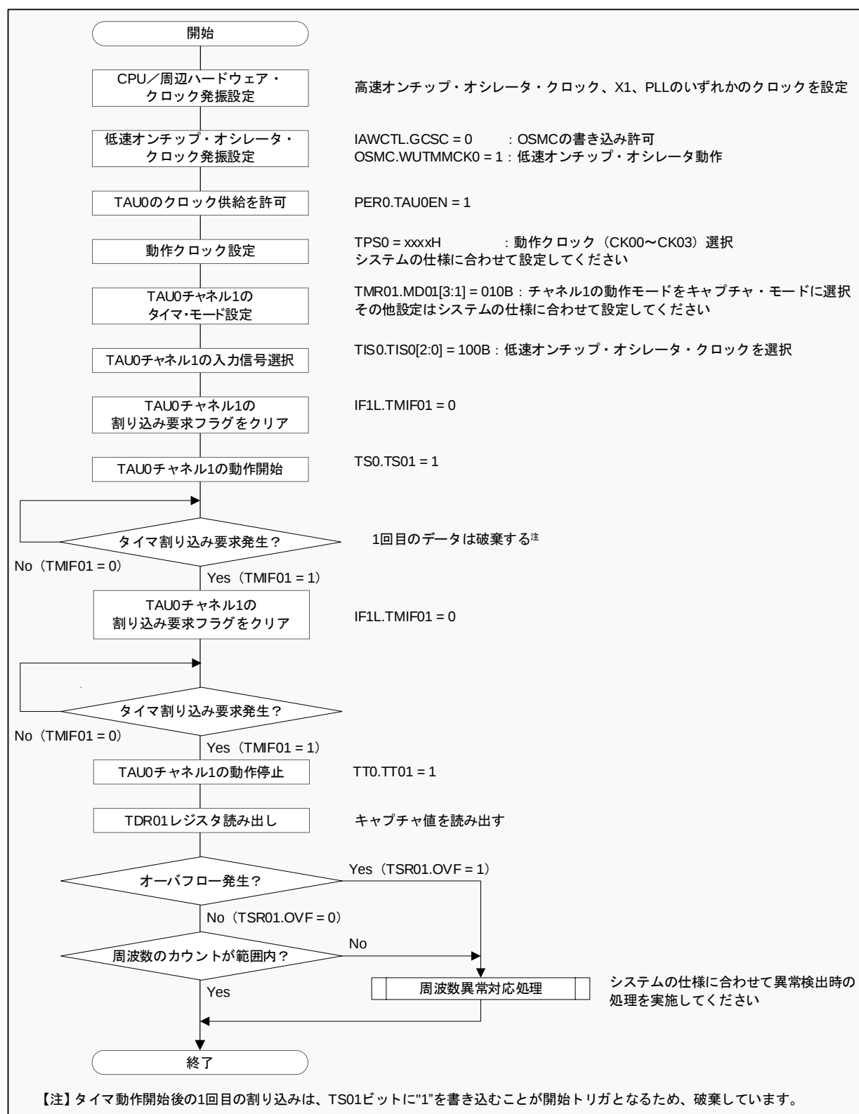
図 10-1 周波数検出機能の使用例
