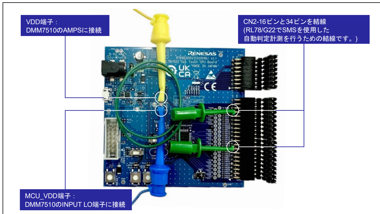
図 7-4 電流計測時の RL78/G22 CPU ボードの配線図
