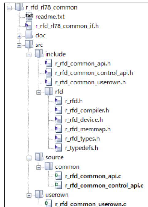
展開時の r_rfd_rl78_common フォルダ
