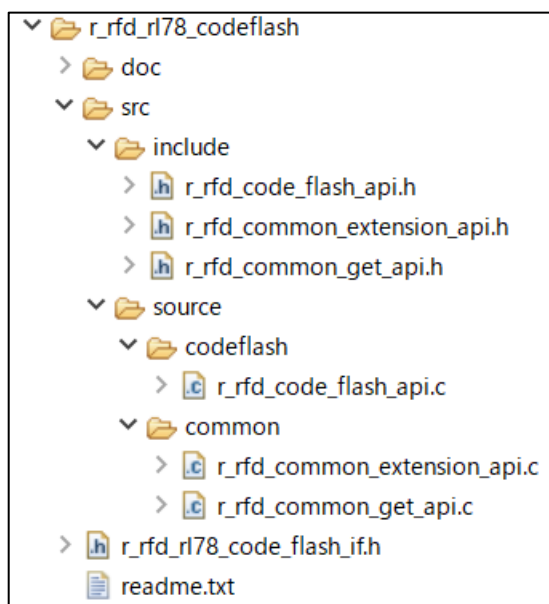
展開時の r_rfd_rl78_codeflash フォルダ
