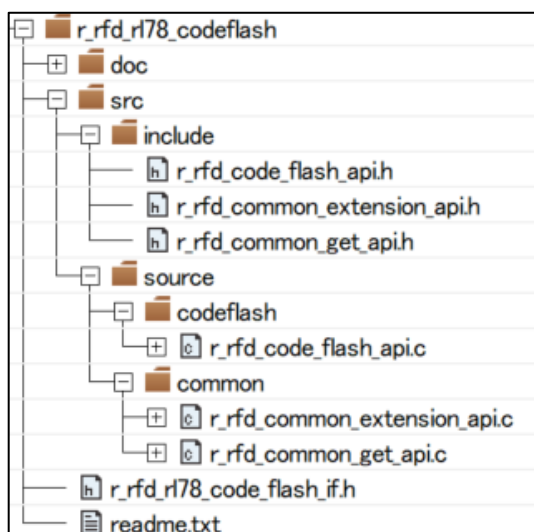
展開時の r_rfd_rl78_codeflash フォルダ
