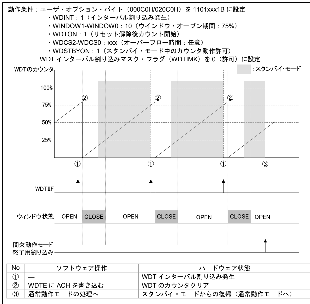
図 2-1 WDT の機能を使用した場合の処理例
