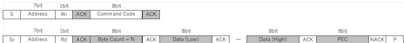
図 1-8 通信フォーマット Block Read
