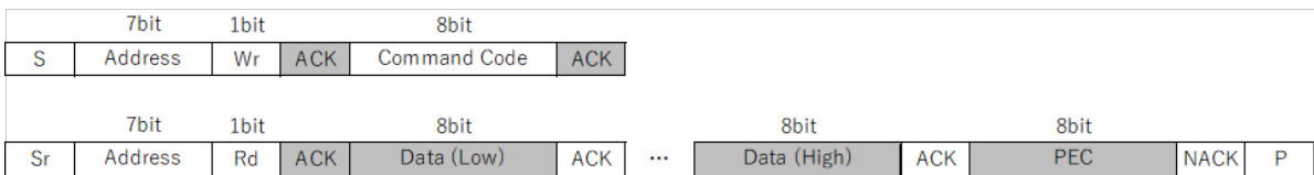
図 4-8 通信フォーマット Read (Multi byte)
