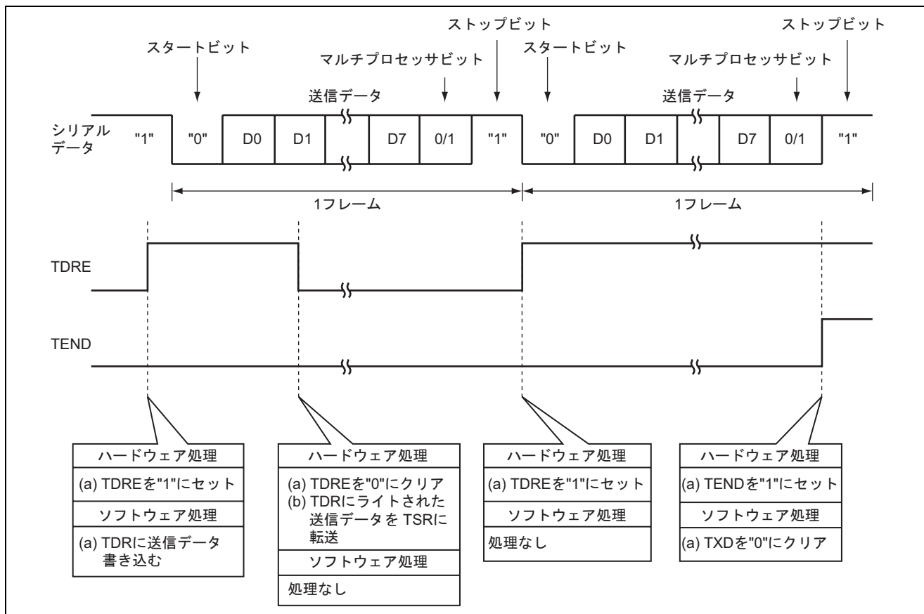
図4 マルチプロセッサ通信機能による送信の動作原理
