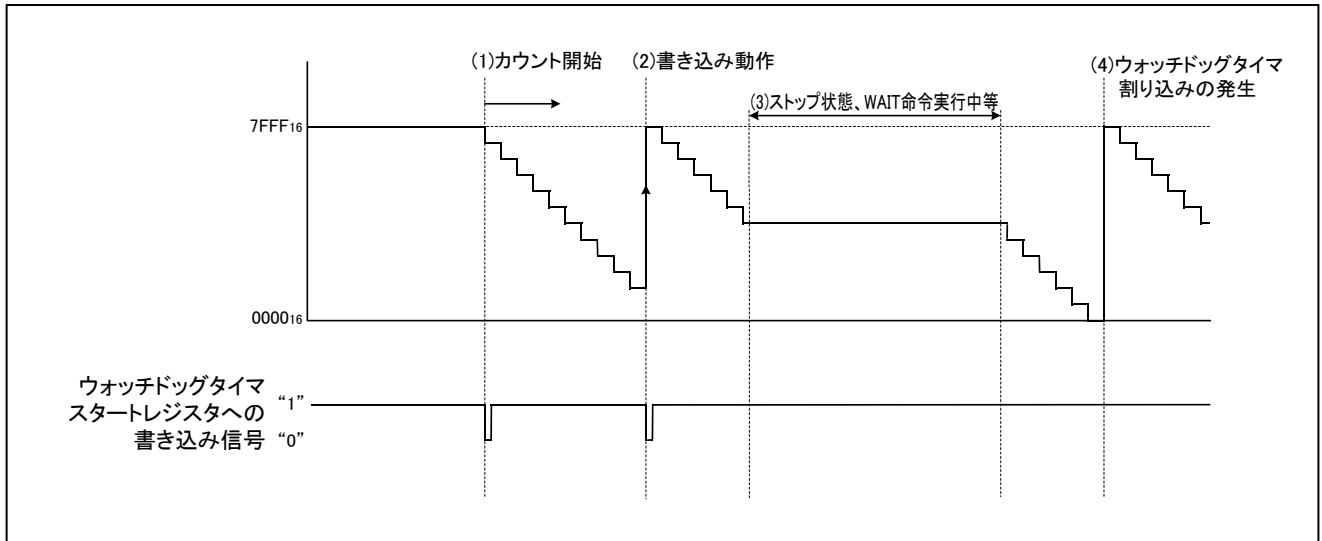
図 1 ウォッチドッグタイマ動作例
