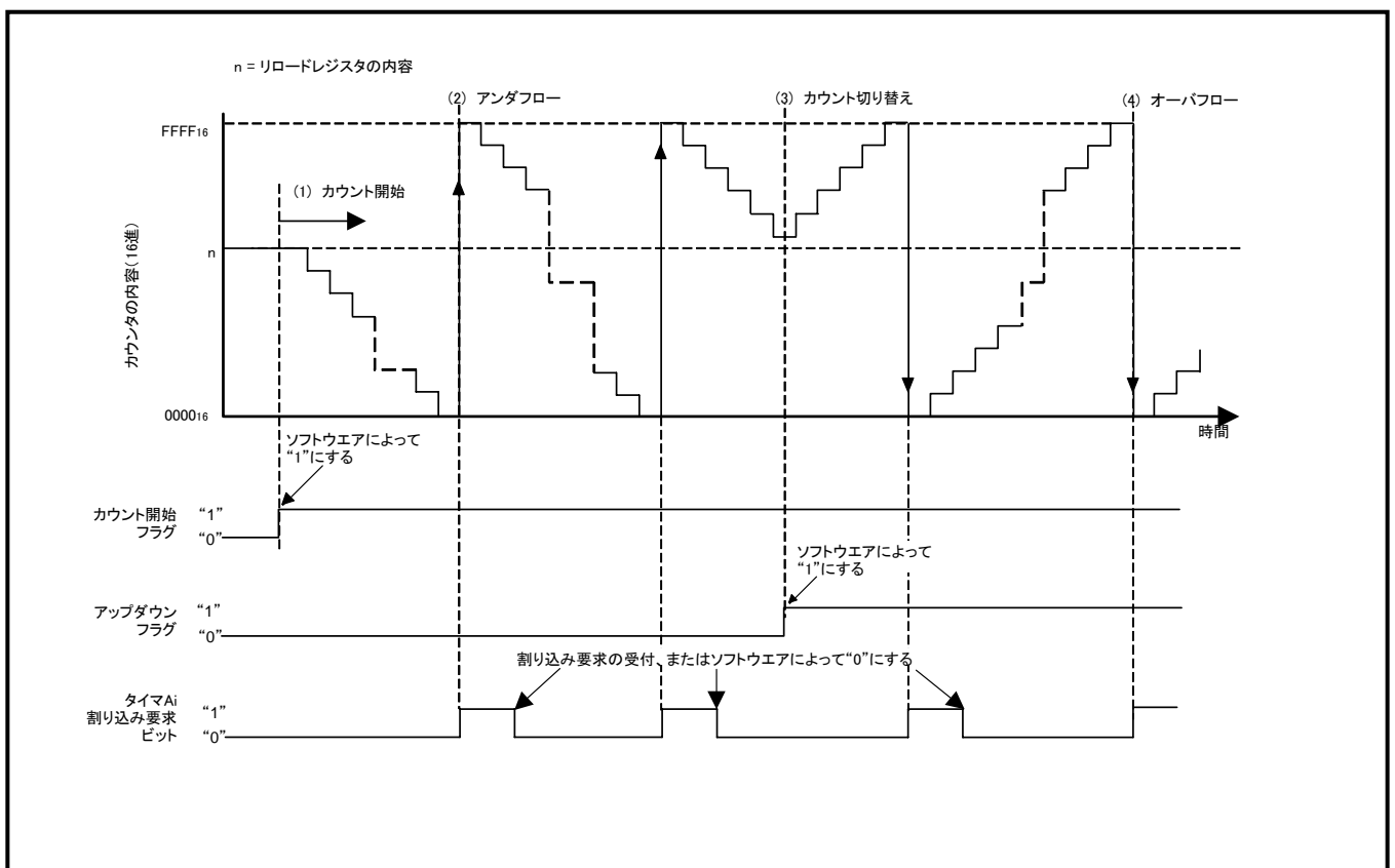
図 1. イベントカウンタモード、フリーランタイプ選択時の動作タイミング図
