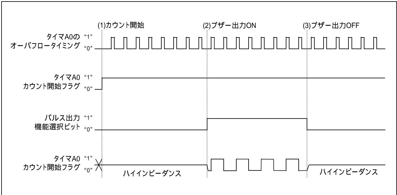
図 1 ブザー出力の動作図
