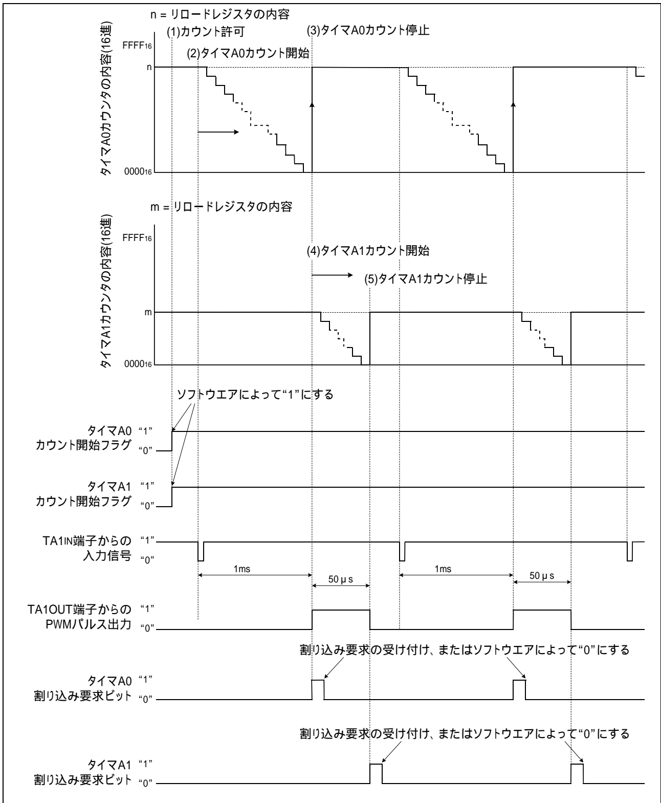
図 1 ディレードワンショット出力動作タイミング
