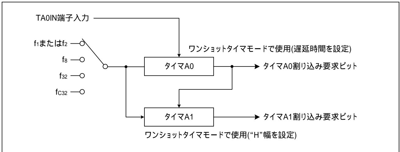
図 2 ディレードワンショット出力のタイマ接続図
