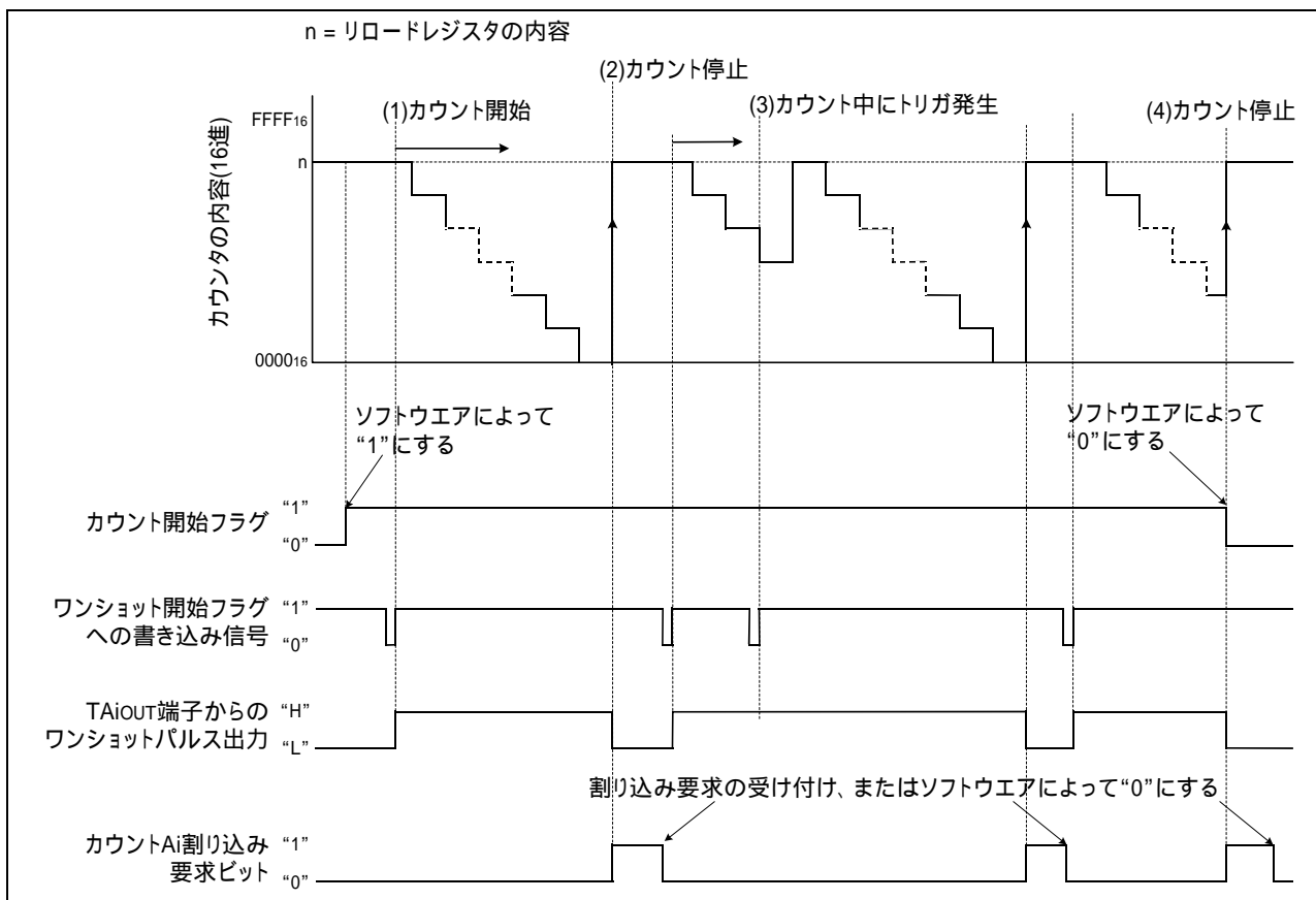
図 1 ワンショットタイマモード動作タイミング
