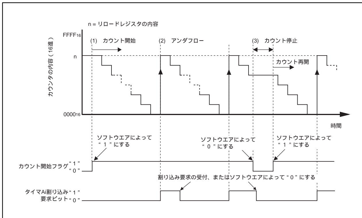
図1 タイマモード動作タイミング
