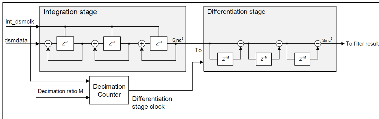
図 2-2 SINC (SINC3) フィルタの概念
