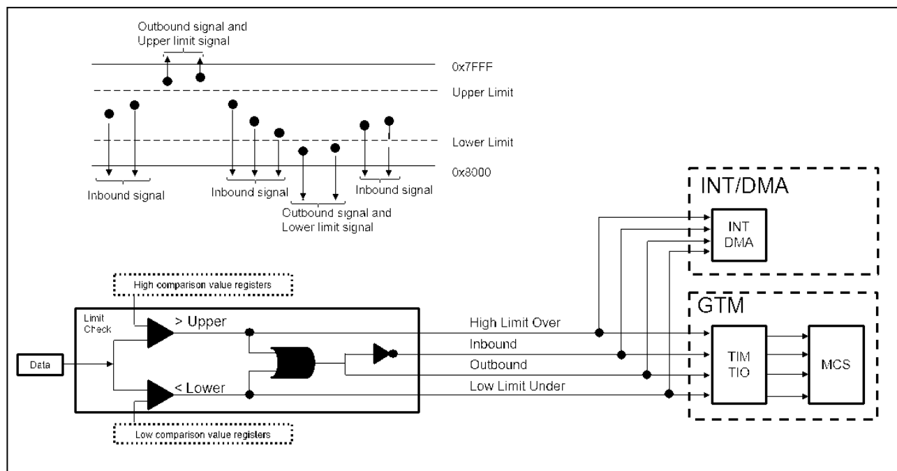
図 2-6 上限値、下限値の検出
