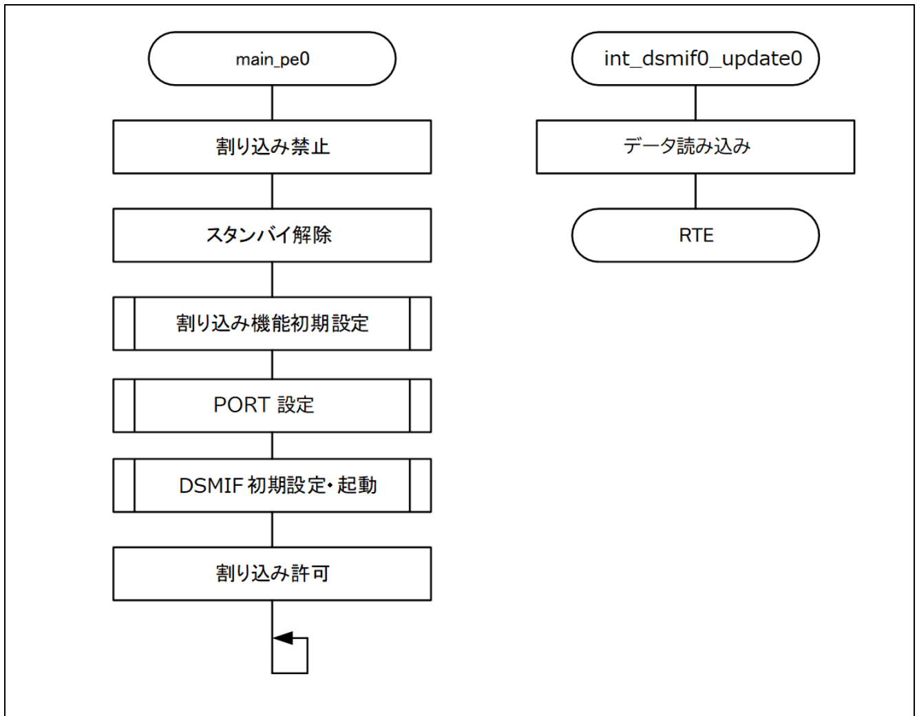
図 3-2 動作フロー
