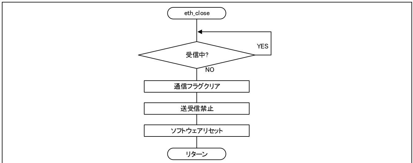
図 1-26 Ether 通信終了モジュールフローチャート
