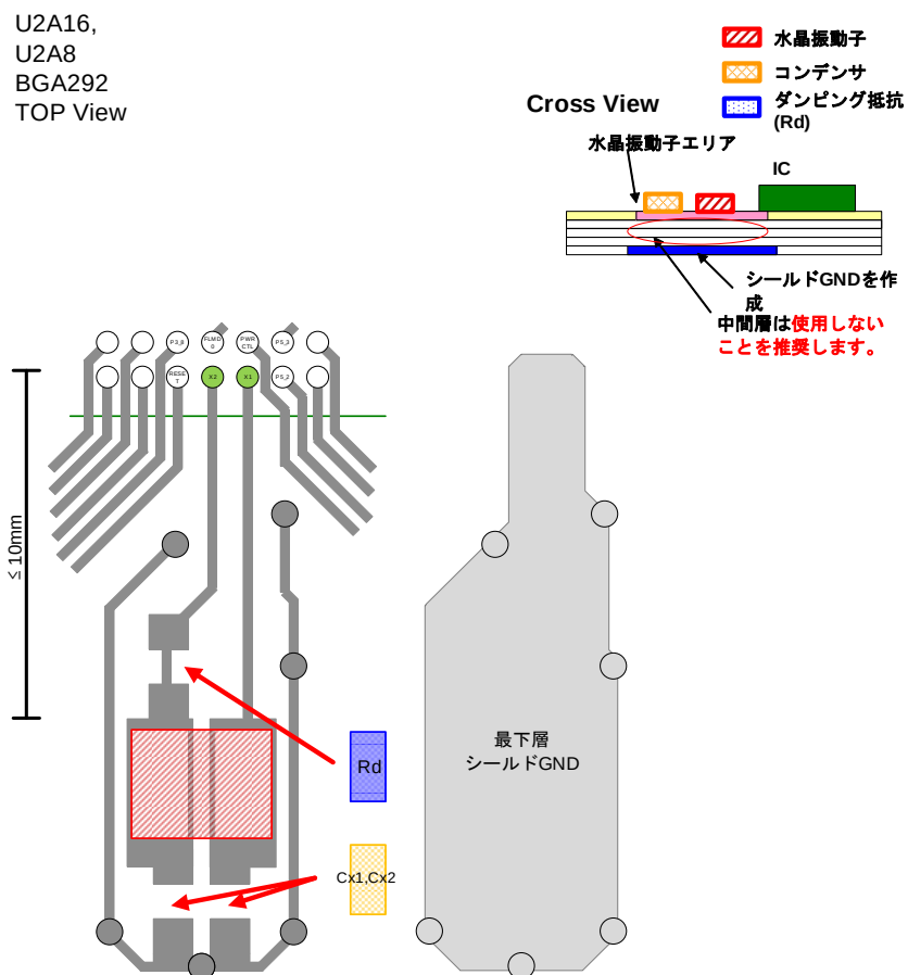
図. 5 安定発振のためのボードパターン例 (U2A16,U2A8 BGA292の場合)
