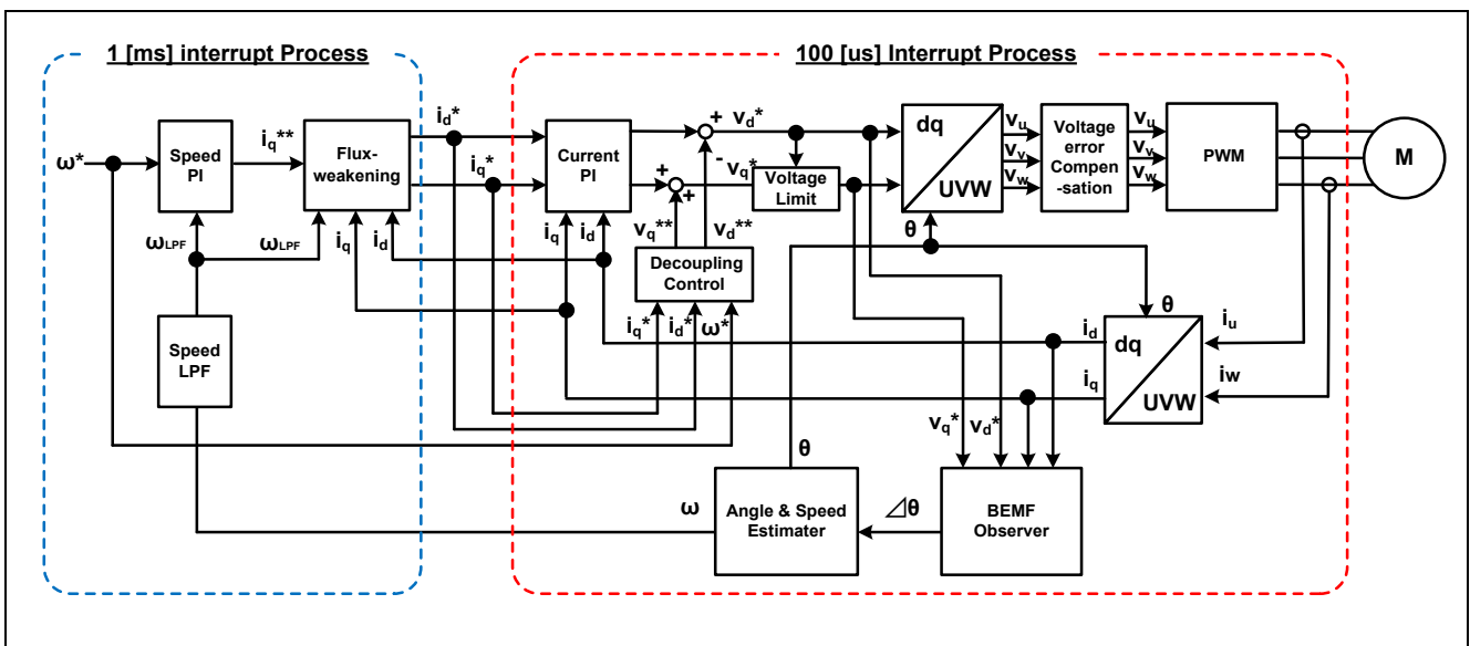
図 3-6 センサレスベクトル制御概略ブロック図(センサレス制御時)
