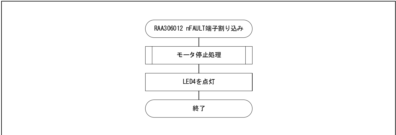
図 3-16 RAA306012 nFAULT 端子割り込み処理フローチャート
