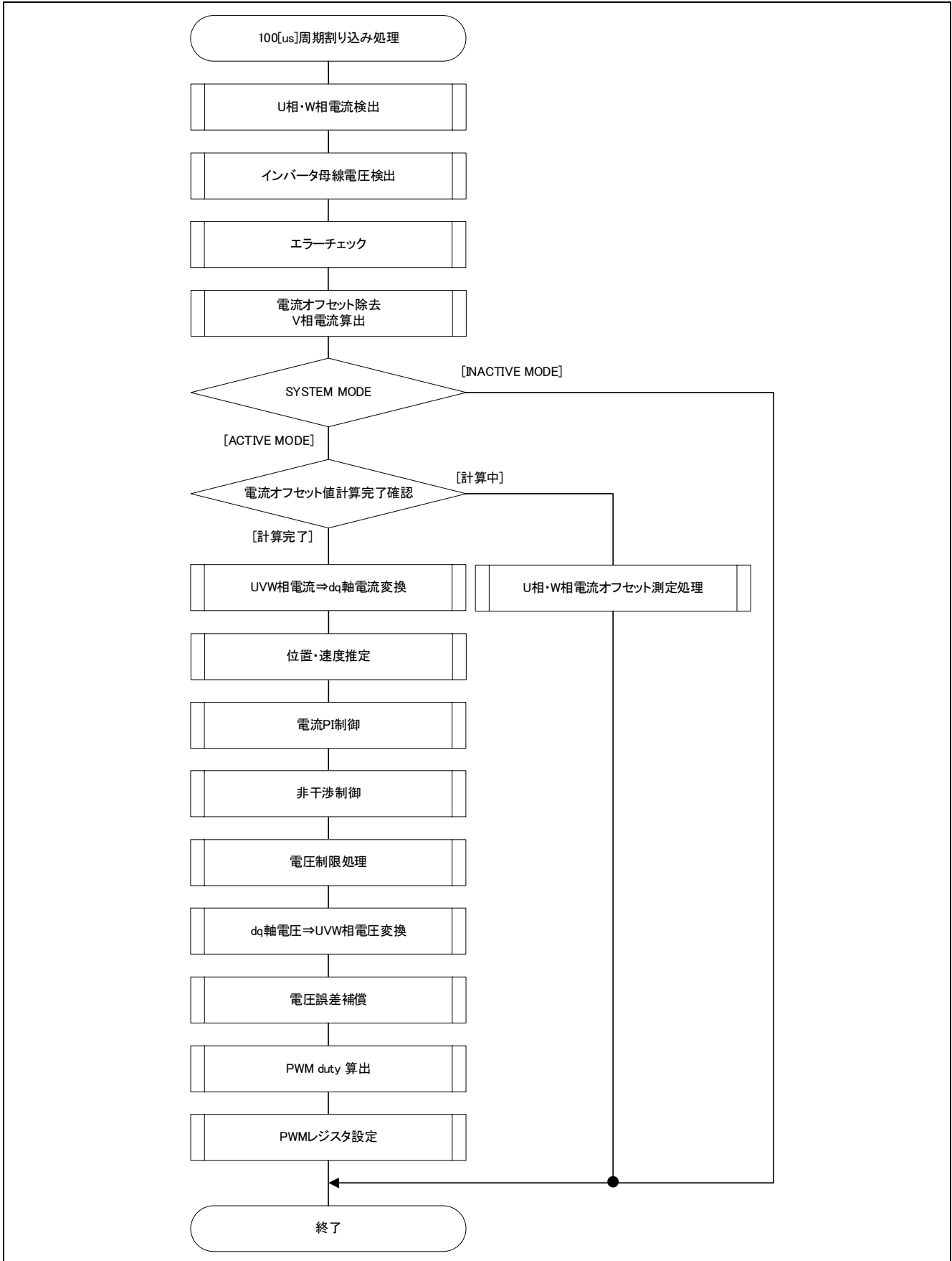
図 3-8 100[μs]周期割り込み処理フローチャート
