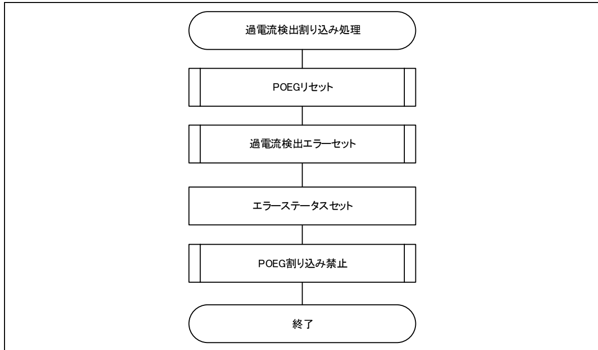
図 3-20 過電流検出割り込み処理フローチャート
