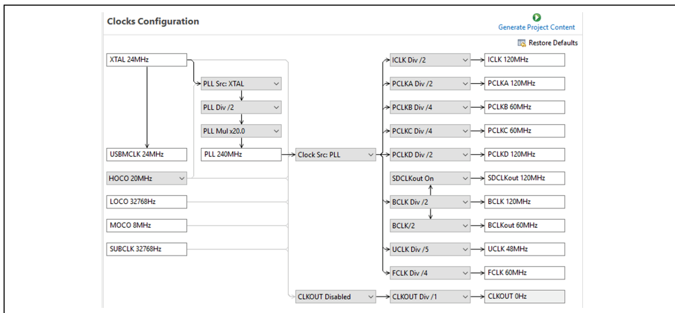
図 11. ルネサス FSP コンフィギュレータによるクロック設定
