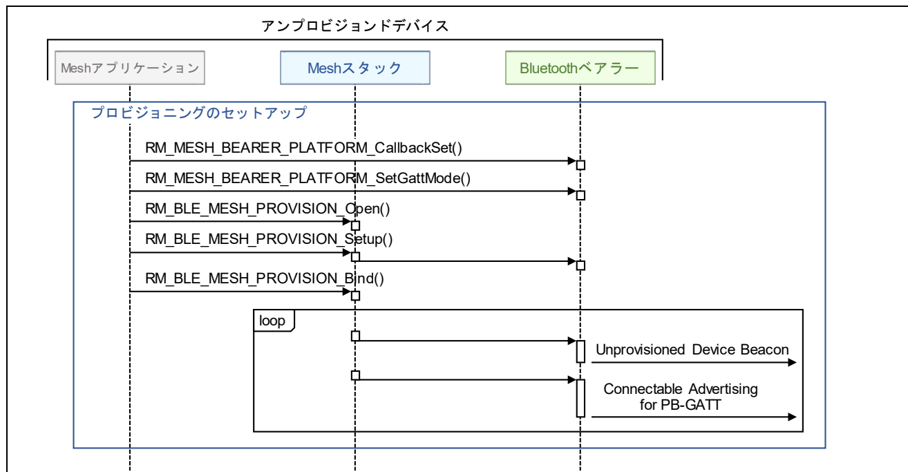
図 3-2 プロビジョニングのセットアップ
