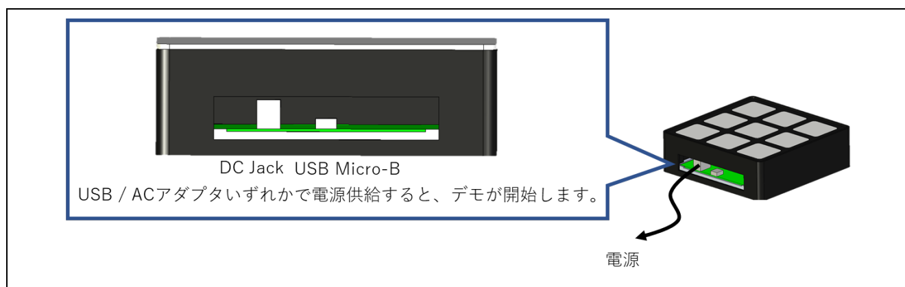
図 2-1 機器接続図
