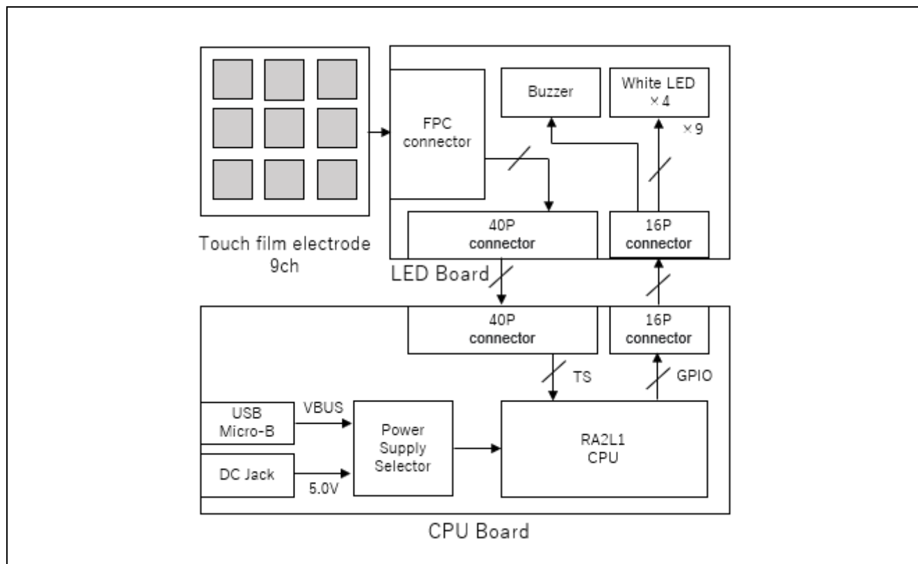
図 4.1 ブロック図
