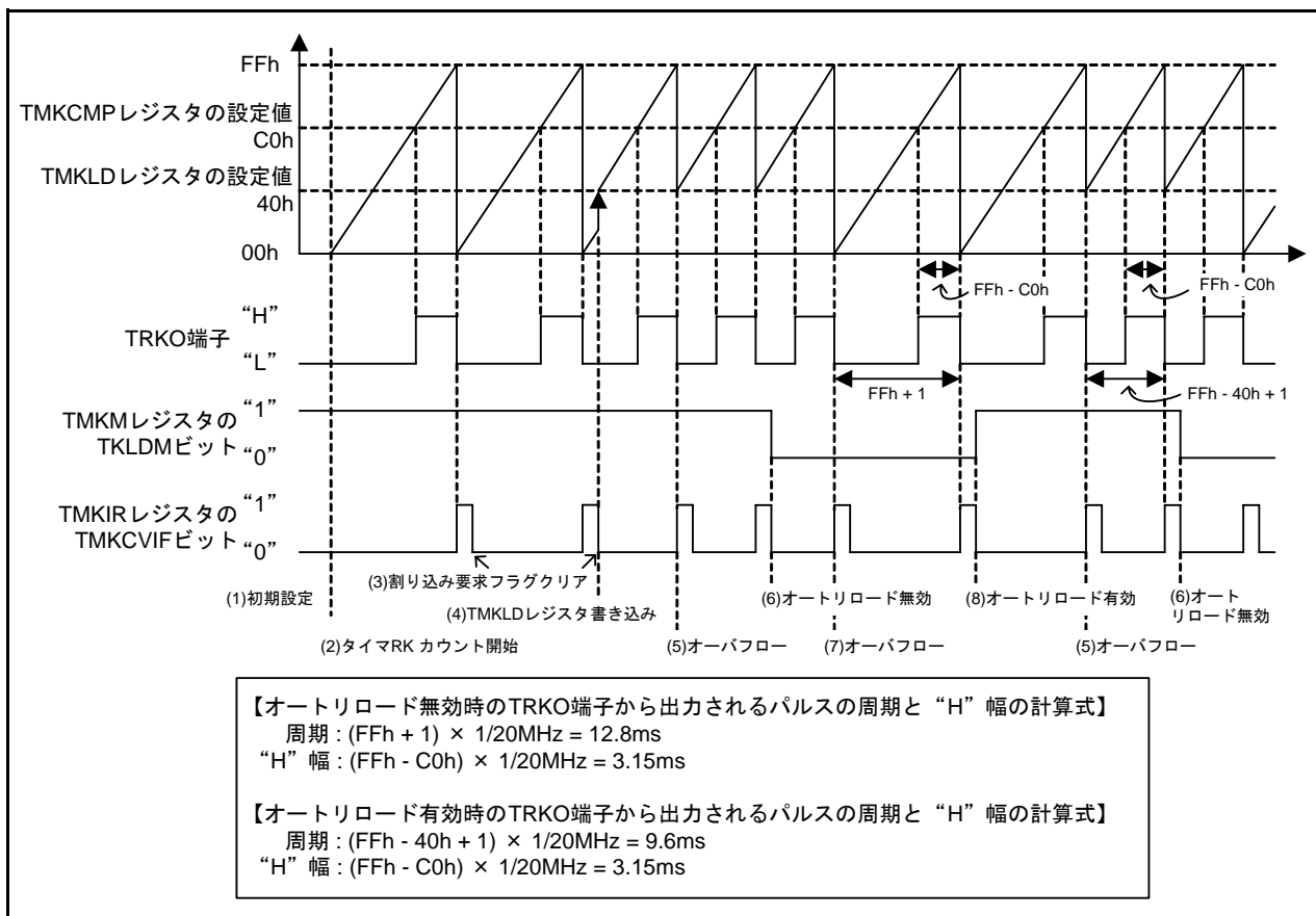
図 4.1 タイミング図
