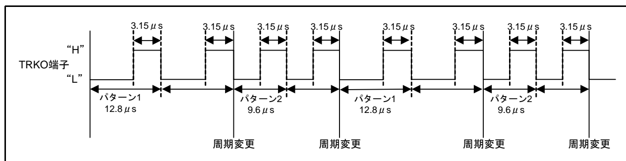
図 1.1 出力波形図
