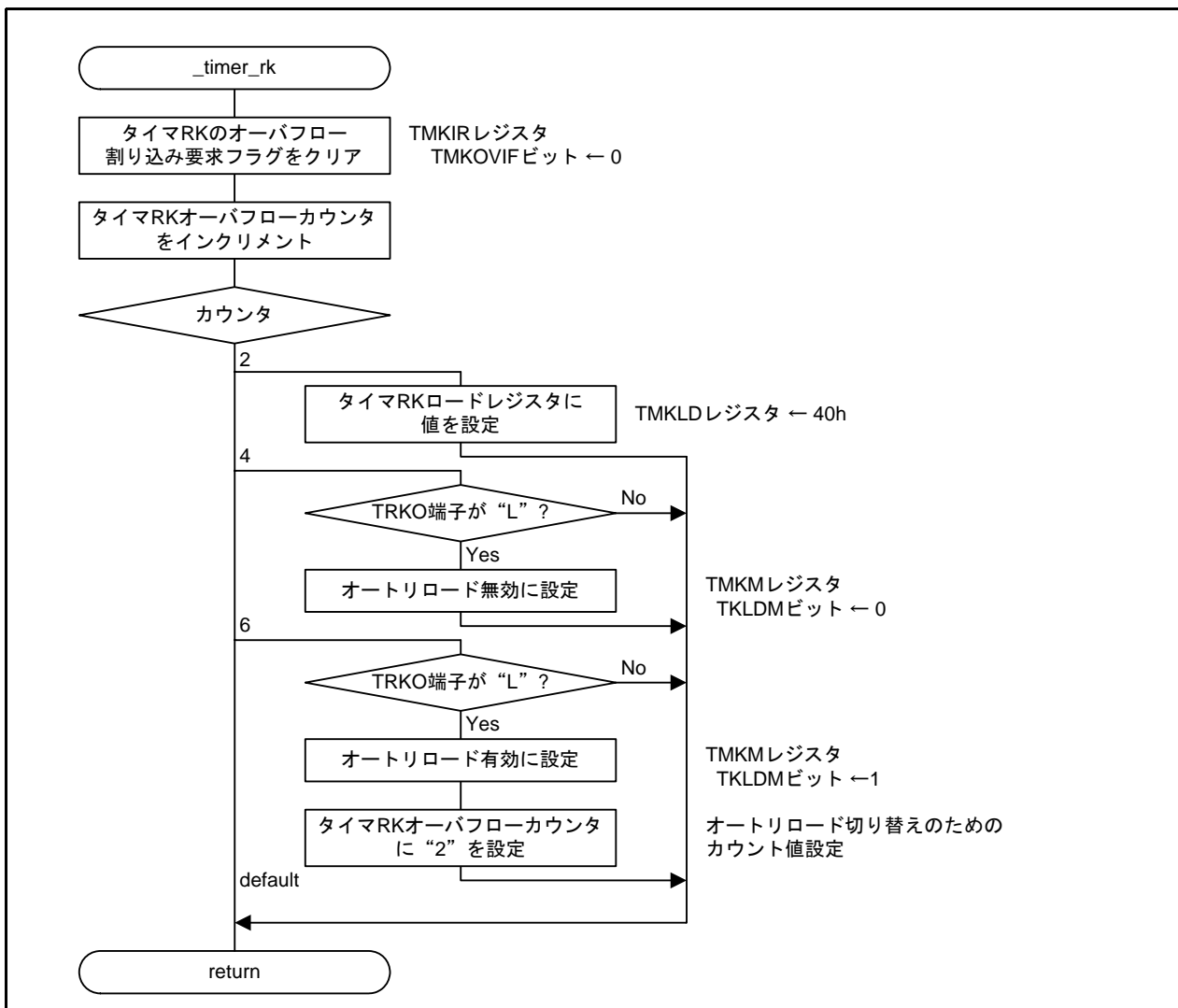
図 4.5 タイマRK割り込み処理
