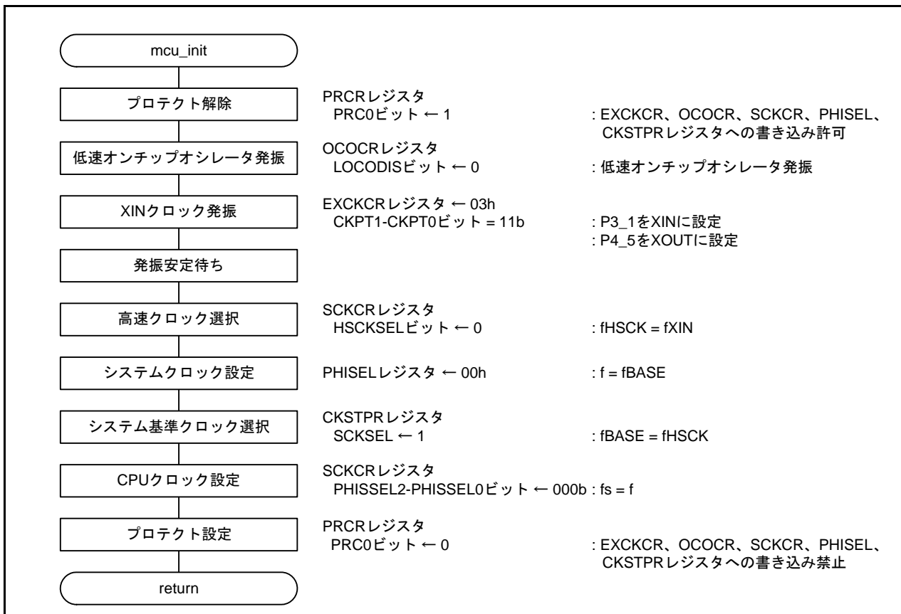
図 4.3 システムクロック設定処理
