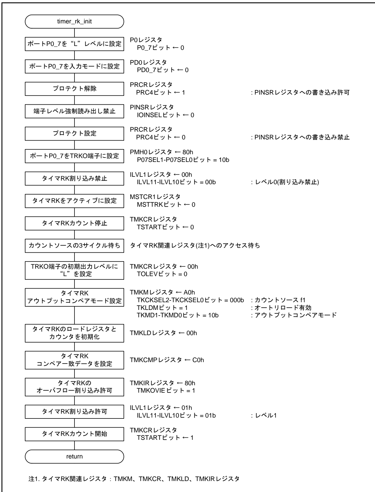
図 4.4 タイマRK初期設定処理
