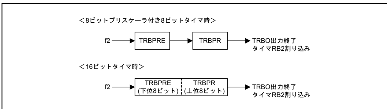
図 3.1 ブロック図
