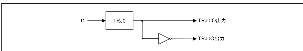
図 3.1 ブロック図
