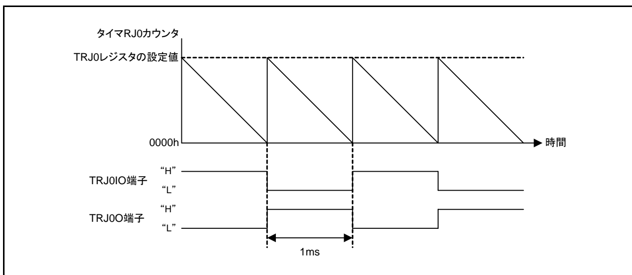
図 3.2 タイミング図
