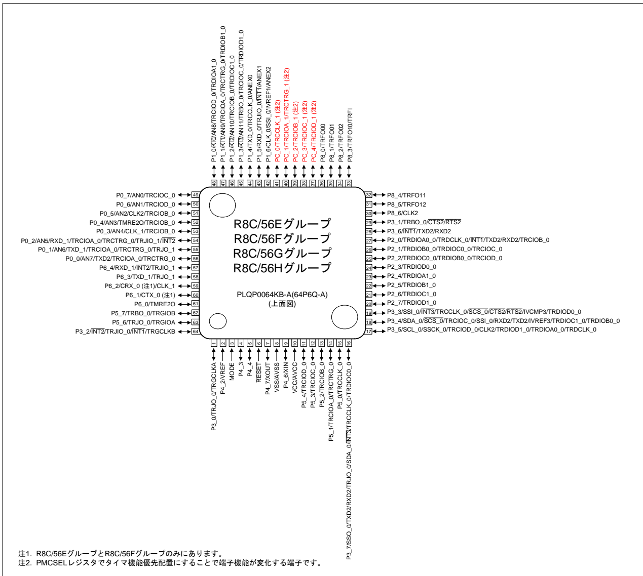
図 1.2 タイマ機能優先端子配置時のピン配置図 (PMCSEL1、PMCSEL0=01b)
