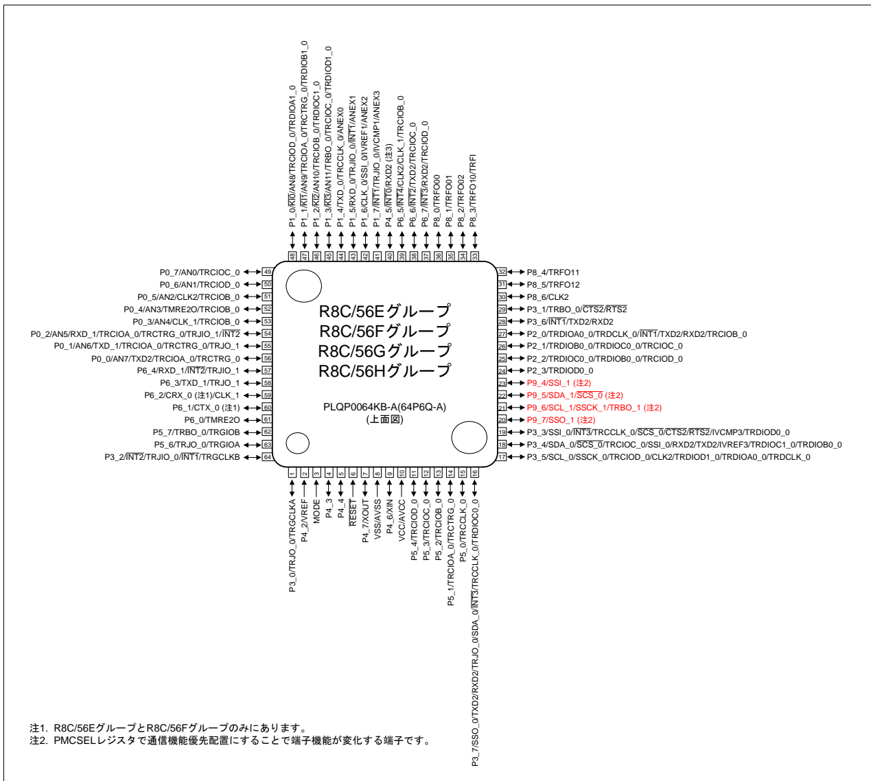
図 1.3 通信機能優先端子配置時のピン配置図 (PMCSEL1、PMCSEL0=10b)
