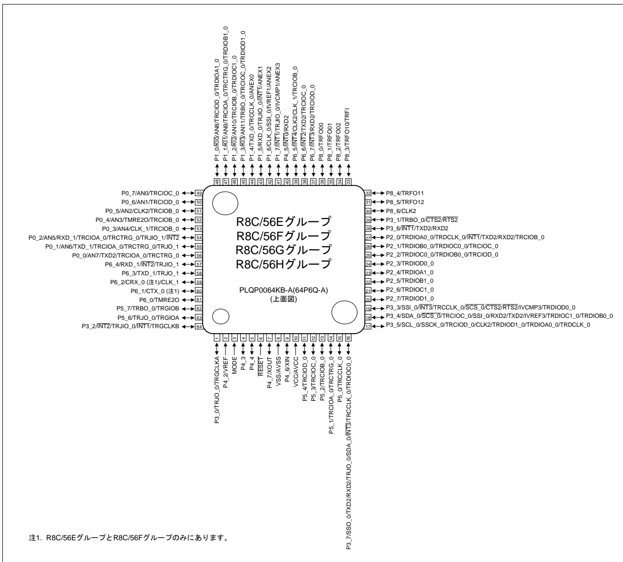
図 1.1 標準端子配置時のピン配置図 (PMCSEL1、PMCSEL0=00b)
