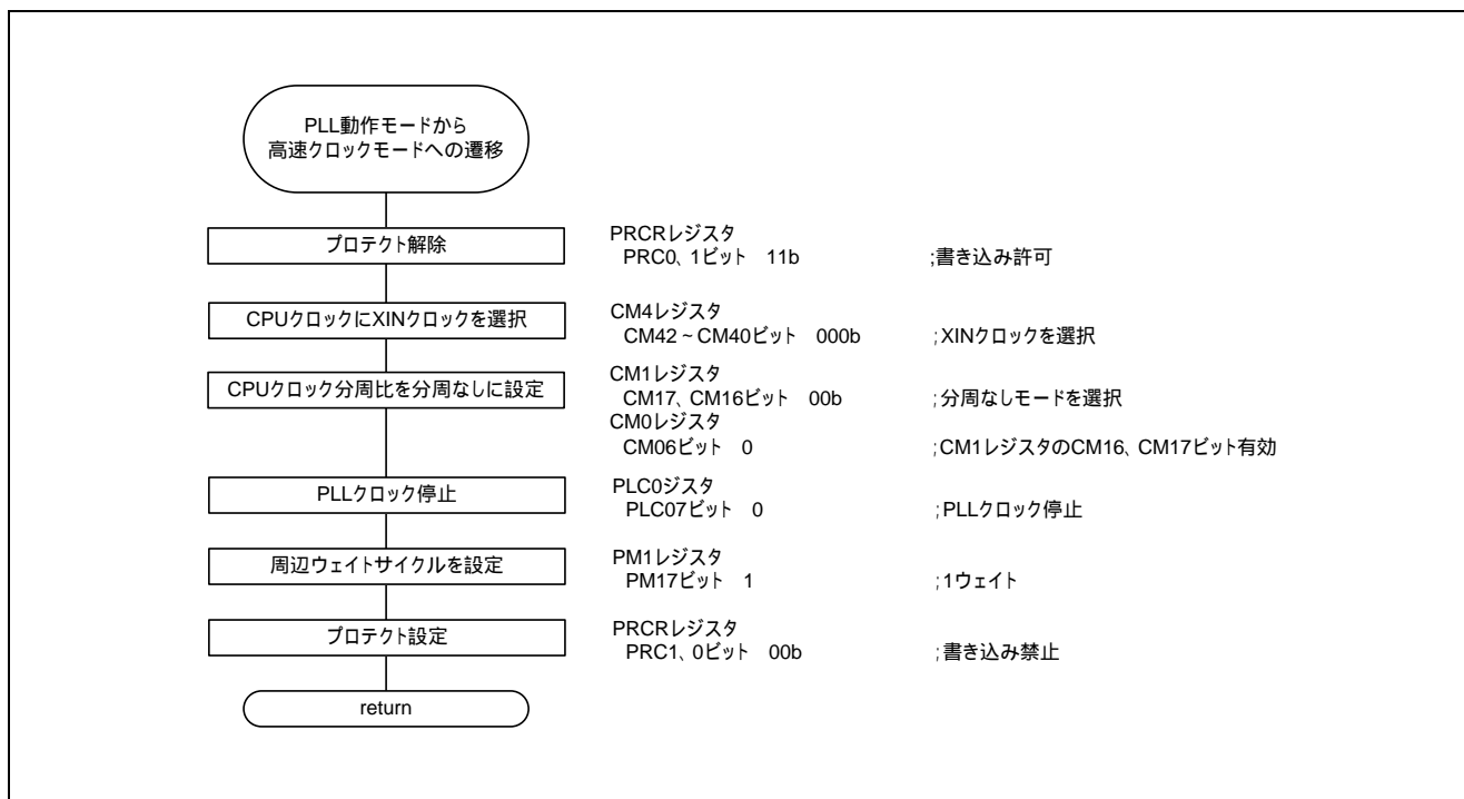
図 1.2 PLL 動作モードから高速クロックモードへの遷移
