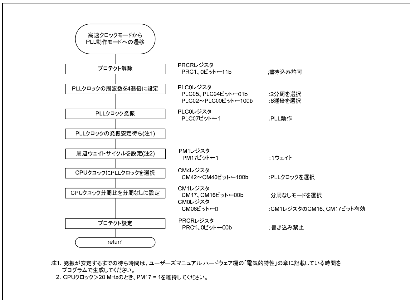
図 1.1 高速クロックモードから PLL 動作モードへの遷移
