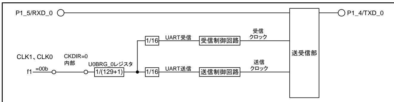
図1.1 ブロック図
