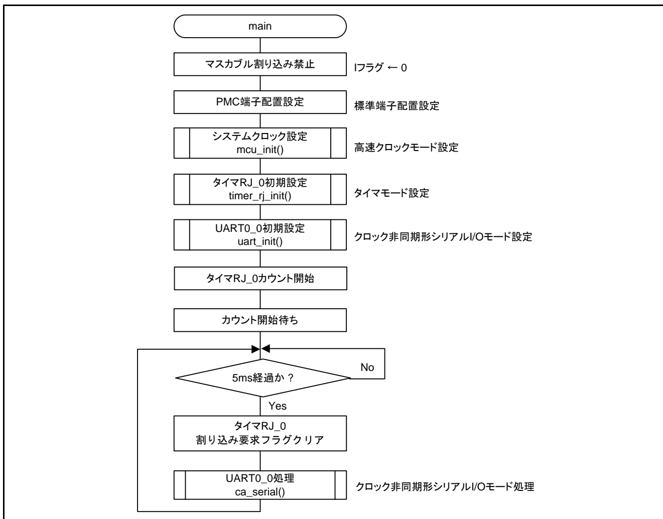
図3.2 メイン処理
