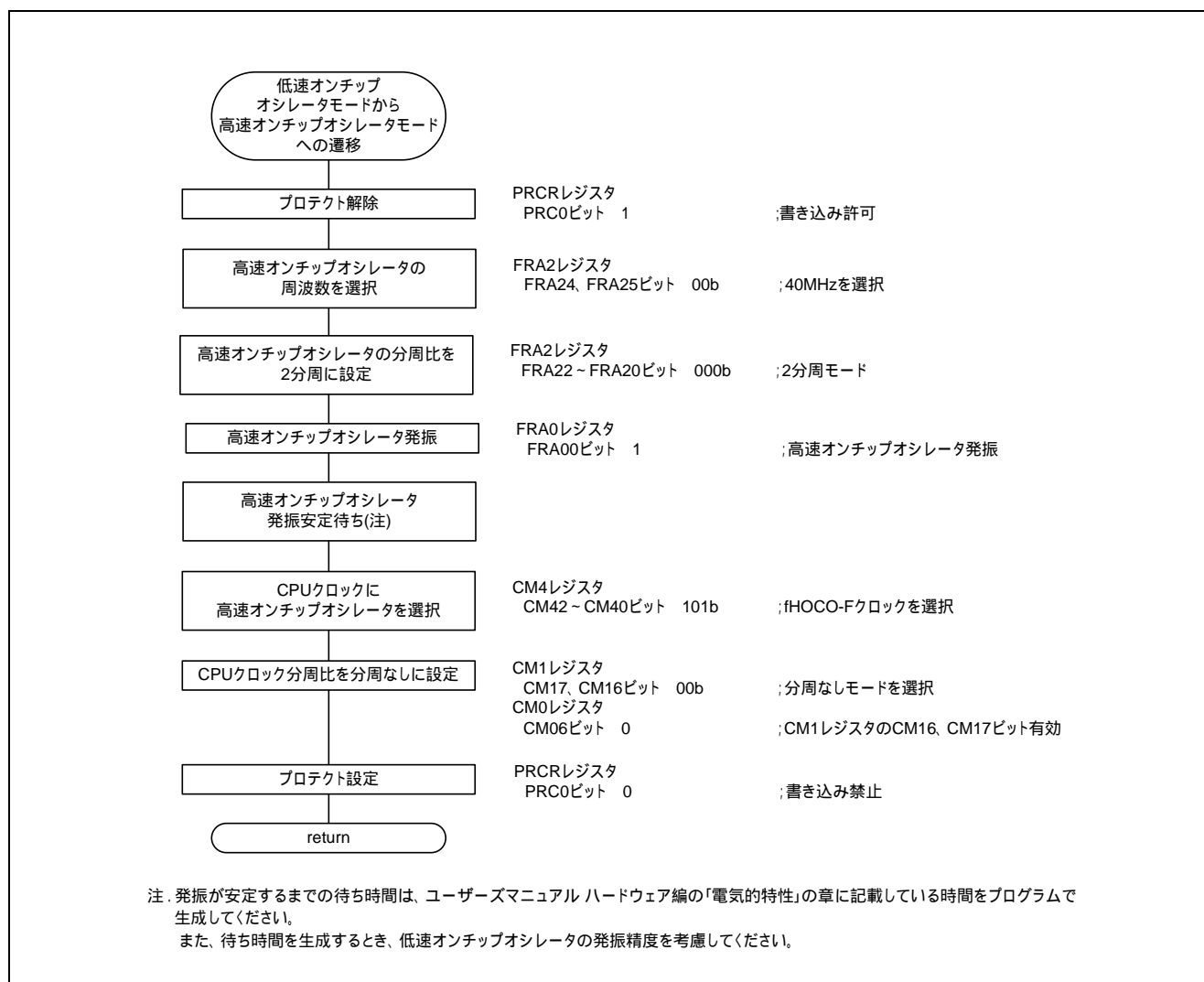
図 1.1 低速オンチップオシレータモードから高速オンチップオシレータモードへの遷移
