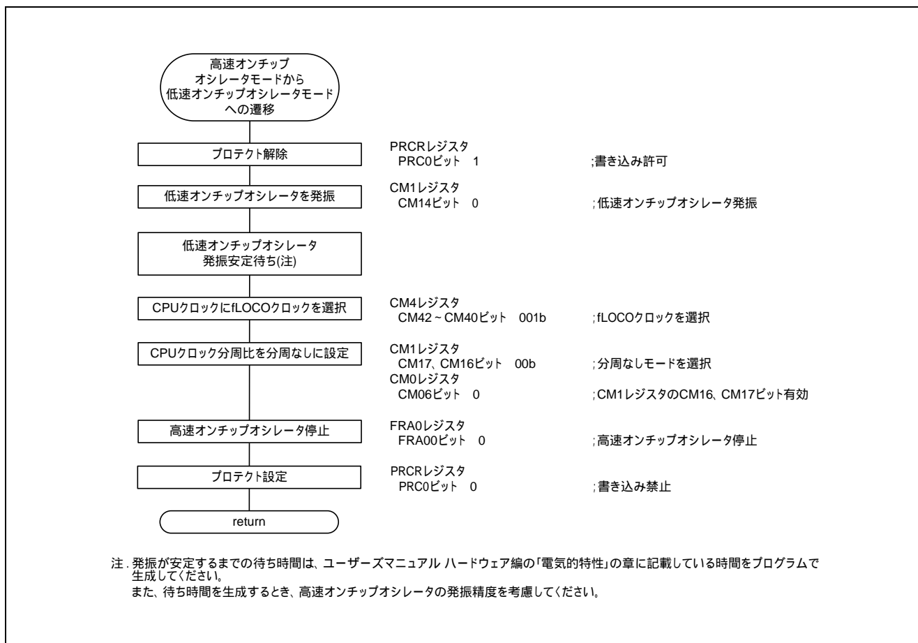
図 1.2 高速オンチップオシレータモードから低速オンチップオシレータモードへの遷移
