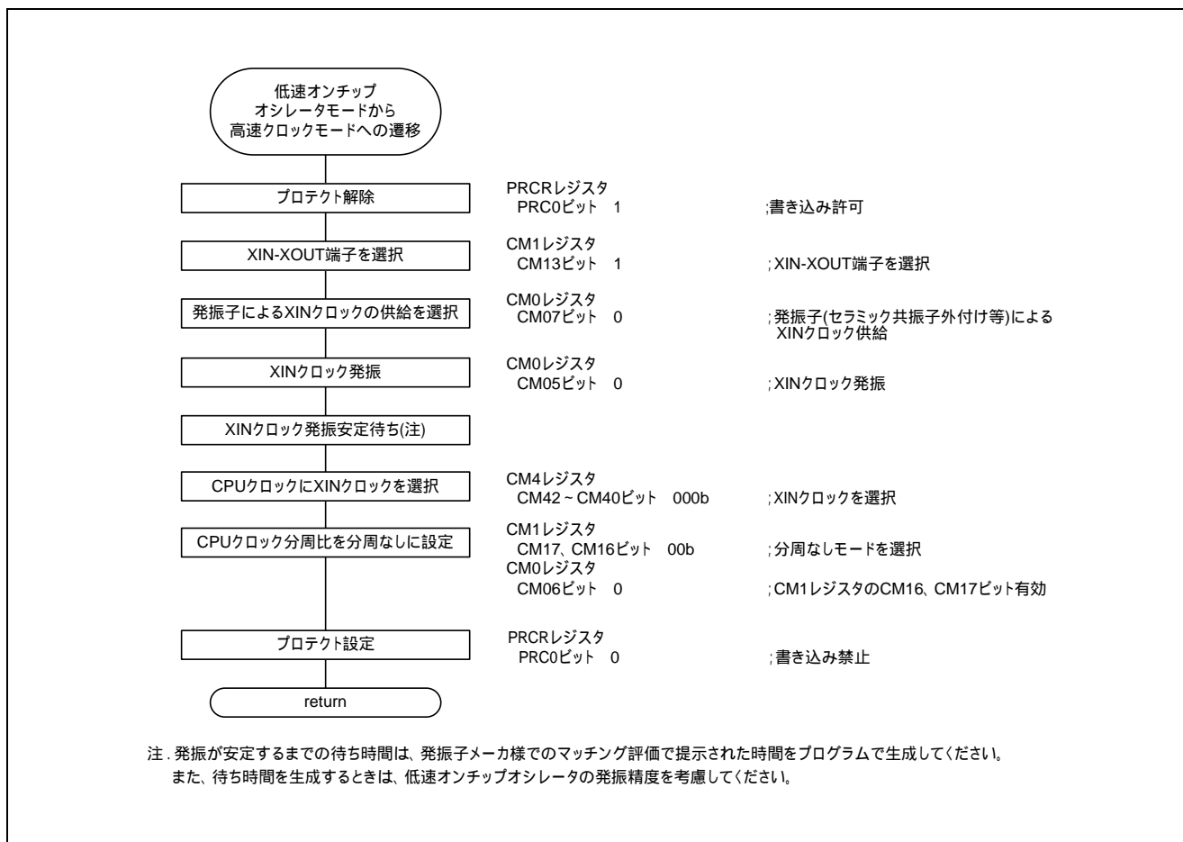
図 1.1 低速オンチップオシレータモードから高速クロックモードへの遷移
