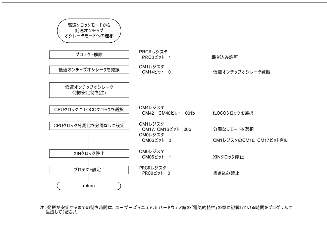
図 1.2 高速クロックモードから低速オンチップオシレータモードへの遷移
