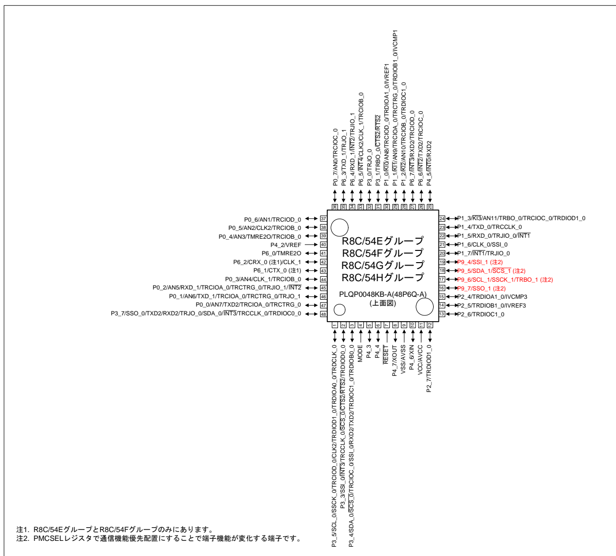
図 1.2 通信機能優先端子配置時のピン配置図 (PMCSEL2~PMCSEL0=100b)
