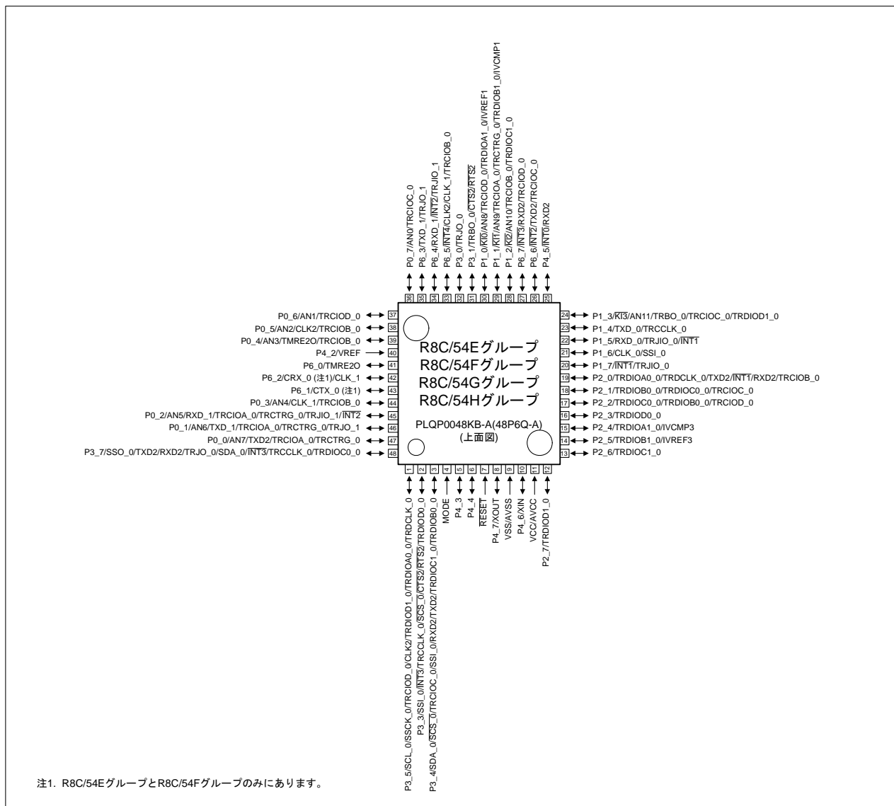
図 1.1 標準端子配置時のピン配置図 (PMCSEL2 ~ PMCSEL0=011b)
