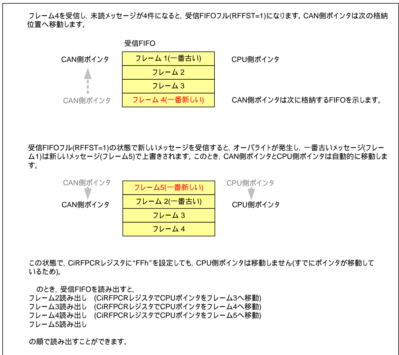
図 1 オーバライトモード時の受信 FIFO ポインタの動作
